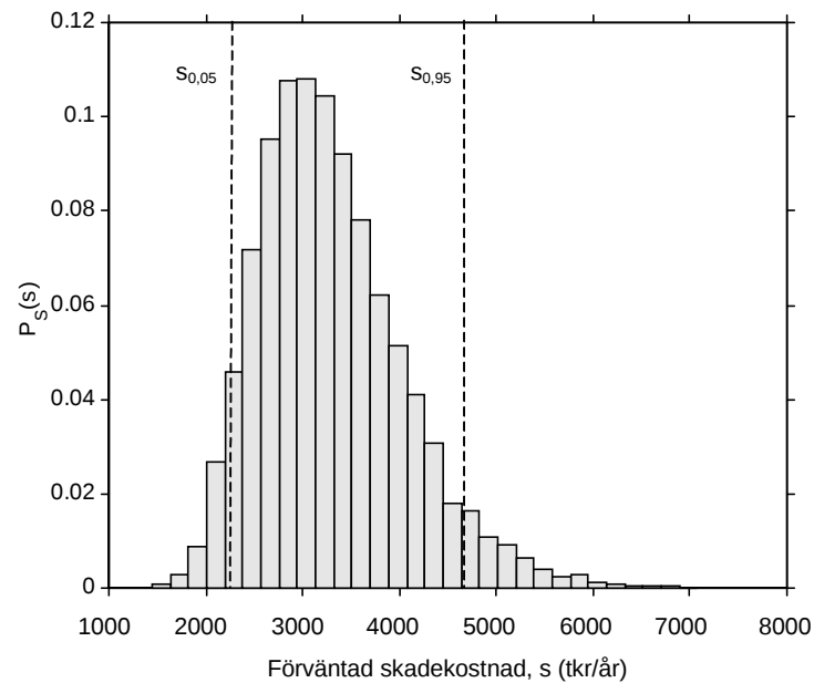
Figur 7 Sannolikhetsfördelningen för den förväntade skadekostnaden i Avesta Sheffield's anläggning.
