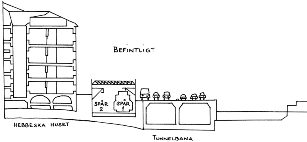
Befintlig spårdragning vid Hebbeska huset (Illustration: H. Corvellec och Angelica Jönsson utifrån Banverkets dokumentation – ej skalenlig).
