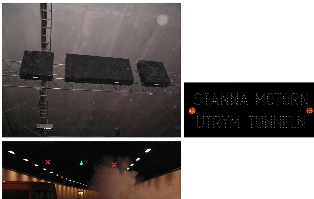
Figur 7. Informationstavla och körfältssignaler i tunneln.
