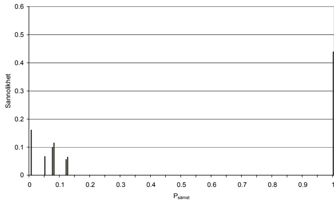
Figur 33. Täthetsfunktionen för P_{sämst} | R > 0 .
