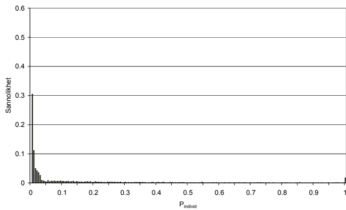
Figur 32. Täthetsfunktionen för P_{individ} | R > 0 .
