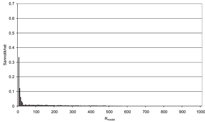
Figur 31. Täthetsfunktionen för R_{medel} | R > 0 .
