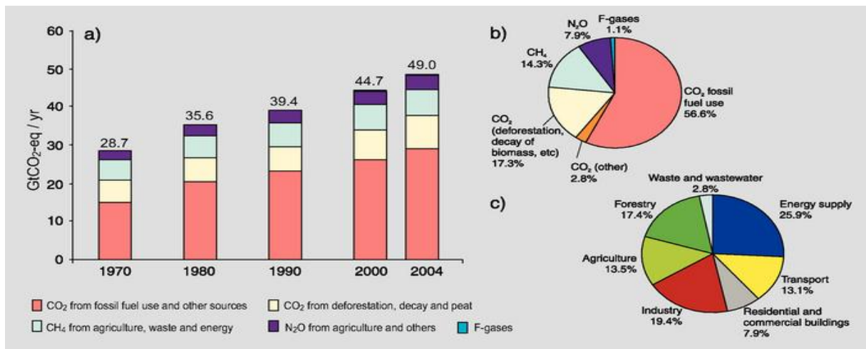
Figur 3: diagrammet visar de antropogena utsläppen av växthusgaser över tiden. Källa www.ipcc.ch/publications_and_data/ar4/syr/en/figure-spm-3.html
