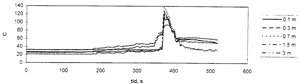
Figur 141. Temperaturträdet försök 7.
