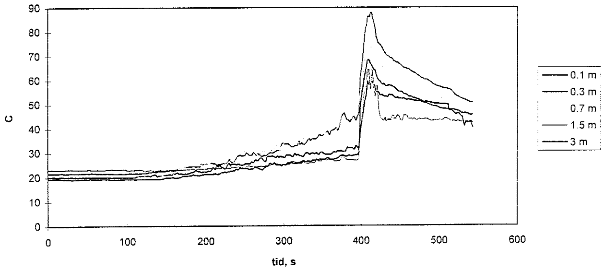
Figur 120. Temperaturträd försök 5.
