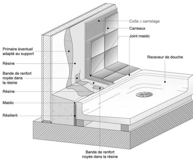
Figur 7.3 Väggen skyddas med primer, tätningsskikt, förstärkningsband vid hörn och kanter, fästmassa och kakelplattor. Primer ska väljas utifrån underlag och är inte obligatorisk. Elastisk fog appliceras vid anslutning till duschbalja.
