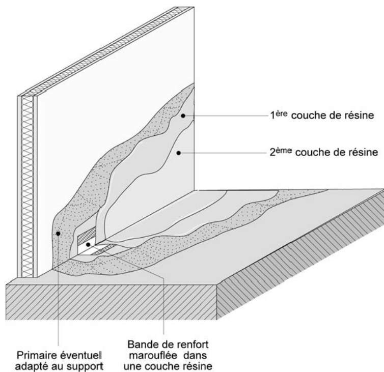
Figur 7.2 Vertikalsnitt som visar anslutning golv-vägg. Keramisk beläggning på både golv och vägg. Två lager tätningsskikt appliceras.
