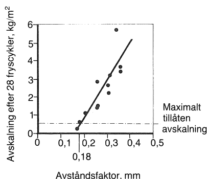
Figur 27. Samband mellan avståndsfaktor och total avskalning efter 28 fryscykler i 3% NaCl-lösning, Fagerlund (1984A).
