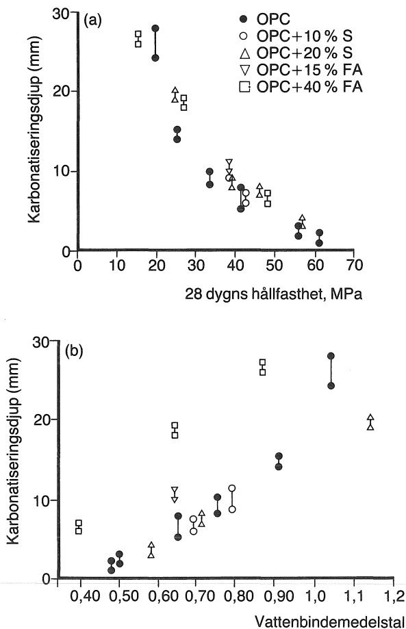
Figur 46. Inverkan av flygaska och silikastoft på karbonatiseringsdjupet hos betong som lagras regnskyddat utomhus, Byfors (1985).
