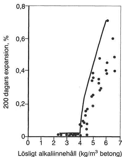
Figur 85. Inverkan av total löslig alkali från portlandcementet på expansionen efter 200 dygn. Hobbs & Gutteridge (1979).
