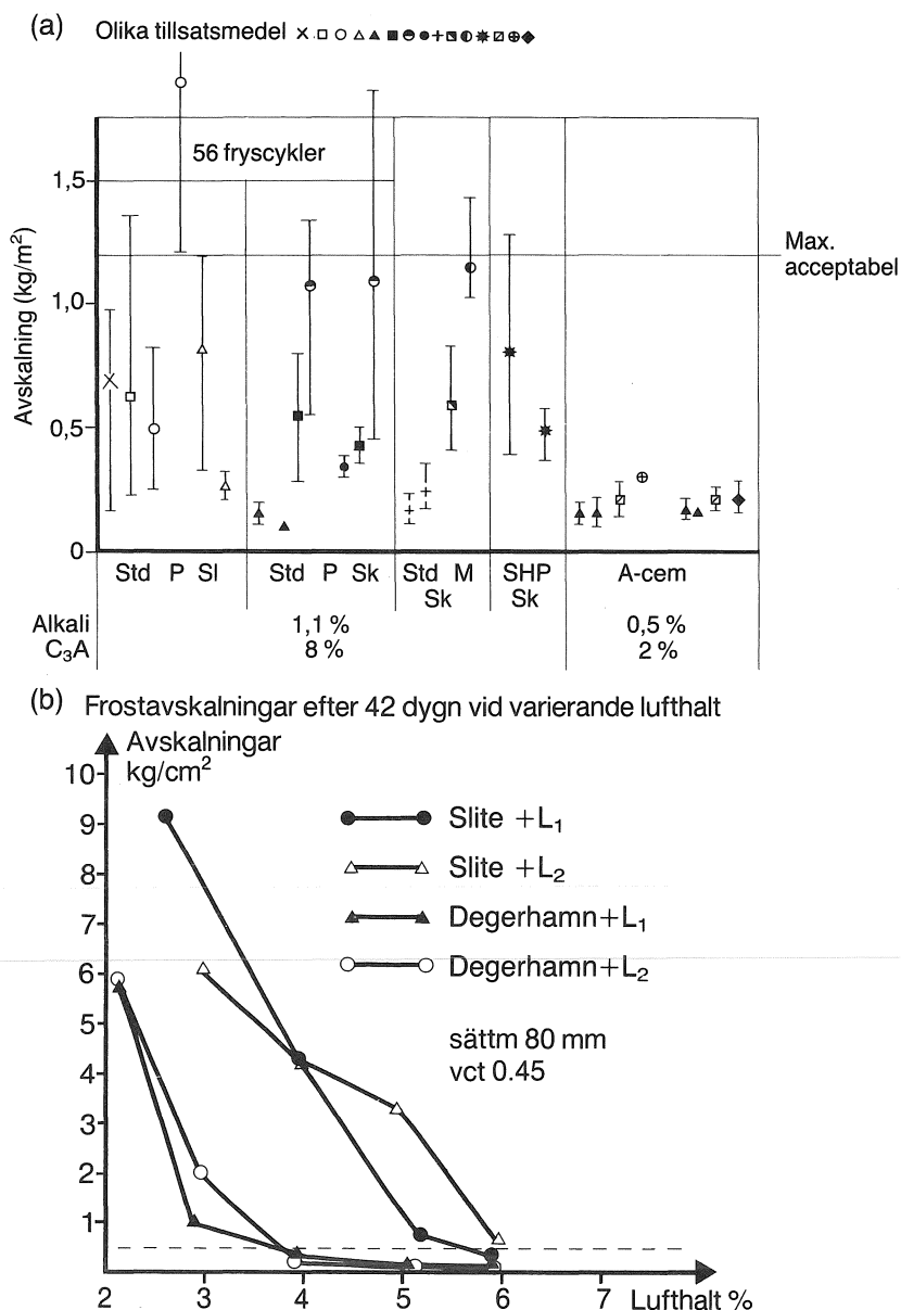
Figur 29. Inverkan av cementsorten på beständigheten vid frysning i 3% natriumkloridlösning.
