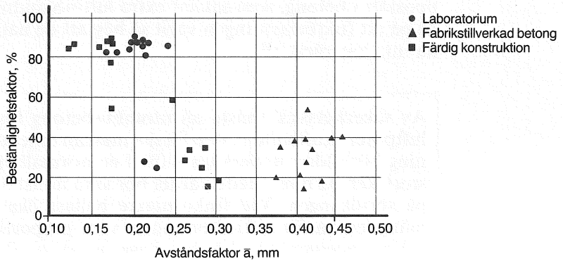
Figur 3. Samband mellan frostbeständighet och avståndsfaktor vid frysning i rent vatten, Ivey & Torrans (1970).
