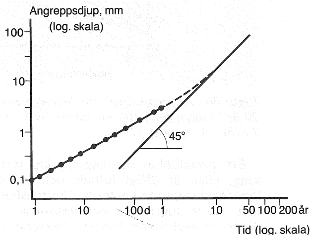
Figur 79. Kemiskt angrepp av saltsyra med pH 3,1 på ett betongrör. På lång sikt följer angreppet troligen linjen med 45°-lutning, Rombén (1979).
