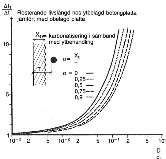
Figur 74. Betong med ytbeläggning. Inverkan av ytskiktets täthet på livslängden. Täckskikt 25mm. (Beträffande beteckningar se ekv (11)). Fagerlund (1984C).
