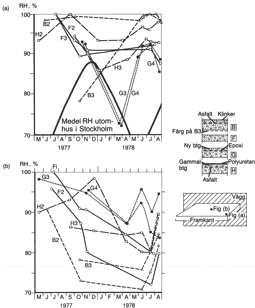
Figur 56. Fuktillstånd i verkliga balkongplattor omedelbart under beläggningen eller omedelbart under betongöverytan, Fagerlund & Svensson (1980).
