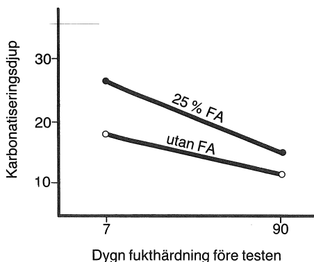
Figur 49. Inverkan av flygaska och fukthärdningstid på karbonatisering av betong med konstant 28-dygnshållfasthet ( f_{28} = 25 MPa). Flygaskhalten (FA) är 20% av total bindemedelshalt. (Accelererad karbonatisering: 4% \text{CO}_2 , 50% RH under 8 veckor). Ho & Lewis (1983).
