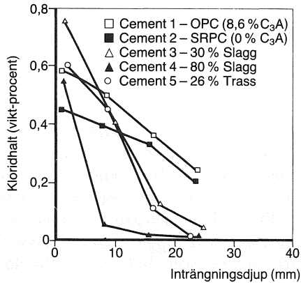
Figur 68. Inverkan av cementtypen på kloridinträngningen vid 6 mån lagring i havsvatten, Gjörv & Vennesland (1979). OPC är portlandcement; SRPC är sulfatresistent portlandcement. Av övriga cement är två slaggcement och ett puzzolancement.
