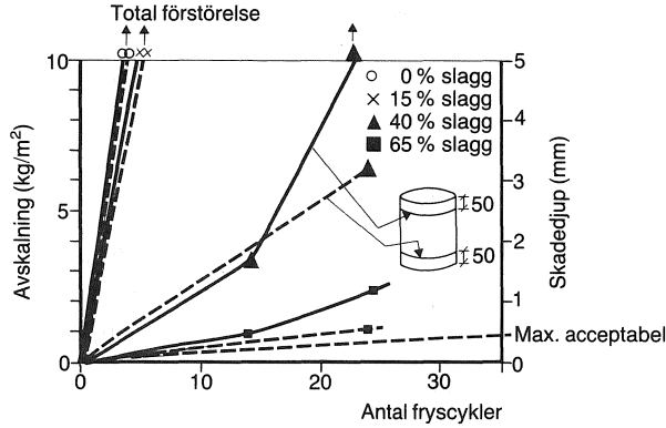
Figur 30. Inverkan av cementets slagghalt på beständigheten vid frysning i 3% natriumkloridlösning. Betong med v_{ct} = 0,45 men utan extra luftinblandning. (2 olika skivor, sågade ur var sin ände av en 200 mm lång cylinder, testades). Fagerlund (1982).
