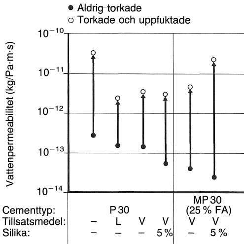
Figur 45. Exempel på inverkan av en uttorknings-uppfuktningscykel på vattenpermeabiliteten. Vattenbindemedelstalet är 0,67 i alla satser, Dahl (1985).
