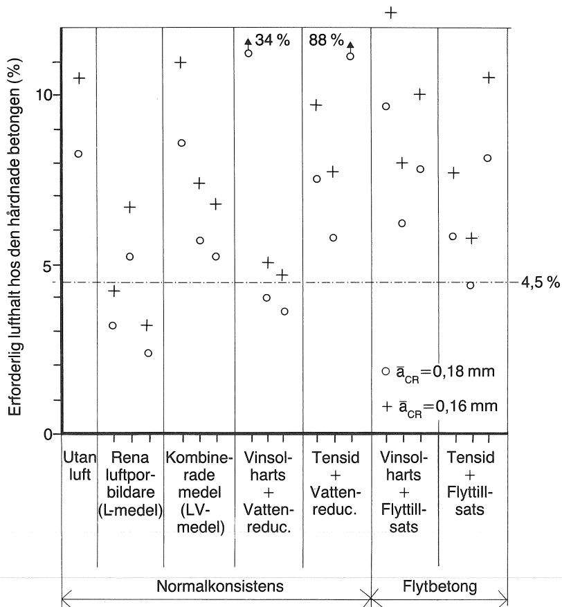
Figur 28. Teoretiskt erforderliga lufthalter hos hård betong beräknade ur luftpordata enligt figur 16 (medelvärden för uppmätta pordiametrar har använts vid beräkningen).
