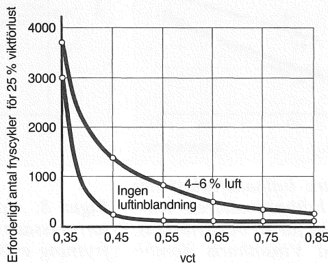
Figur 6. Samband mellan frostbeständighet och vattencementtal, US Bureau of Reclamation (1955).
