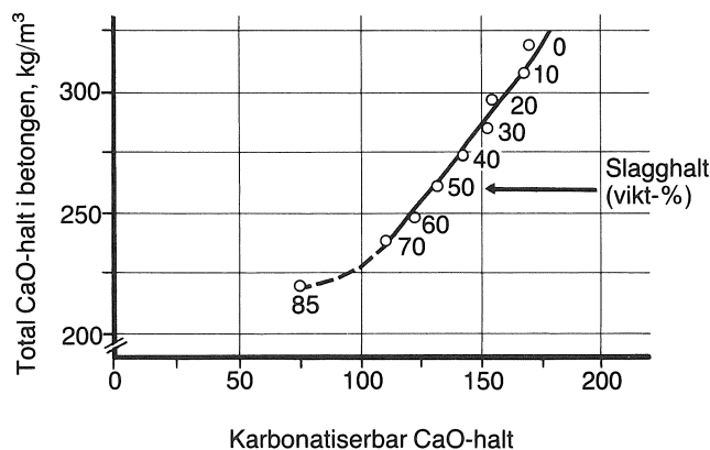
Figur 48. Inverkan av slagghalten hos slaggcementbetong på total kalkhalt och karbonatiserbar kalkhalt, Ludwig (1985).
