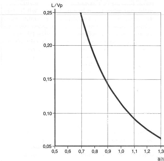
Figur 2. Samband mellan luftpordiameter \bar{D} , cementpastavolym V_p , lufthalt L och luftporavstånd (avståndsfaktor) \bar{a} ; ekv (1).
