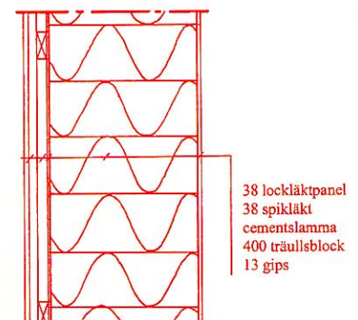
Figur 7. Sektioner av ytterväggs-konstruktionerna: a) högdelen, b) lågdelen. Ovanför fönster och dörrar används armerade träulls-plattor.
