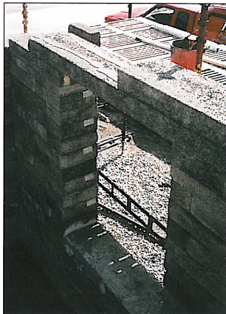
Figur 4. En armerad träullsplatta använd som balk över fönsteröppning.
