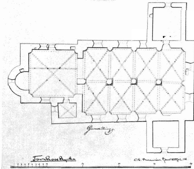
Fig 8. St Thora i Torekov blev skiftevis kaldt kapel og kirke, men afveg iøvrigt ikke fra talrige sognekirker både på landet og i købstæderne. Opmåling af Carl Georg Brunius i Antikvarisk-topografiska arkivet i Stockholm.
