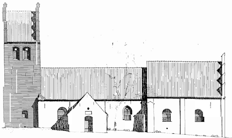
Fig 3. Tibirke kirke. Opmåling af Valdemar Voeler 1926 i Nationalmuseet i København.
