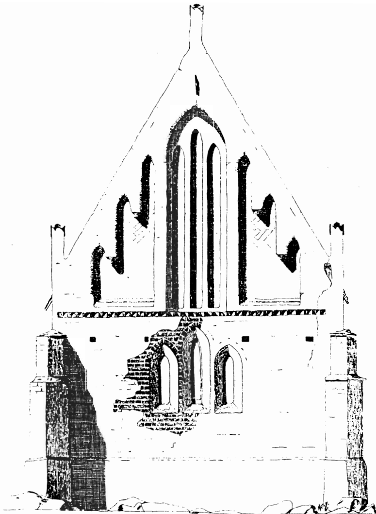
Fig 34. Romansk eller gotisk? Ønslev kirke på Falster, her illustreret med sin korgavl, beskrives trods sine spidsbuede portaler, vinduer og blændinger som senromansk i "Danmarks Kirker". Opmåling ved Eivind Lorenzen 1942 efter DK VIII (1951).
