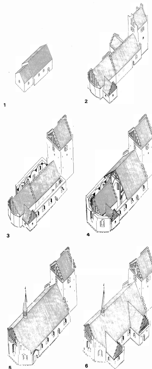
Fig 2. Hovedetaper i Holmstrup kirkes udvikling. Rekonstruk- tioner ved Mogens Vedsø 1988 efter DK IV (1989).
