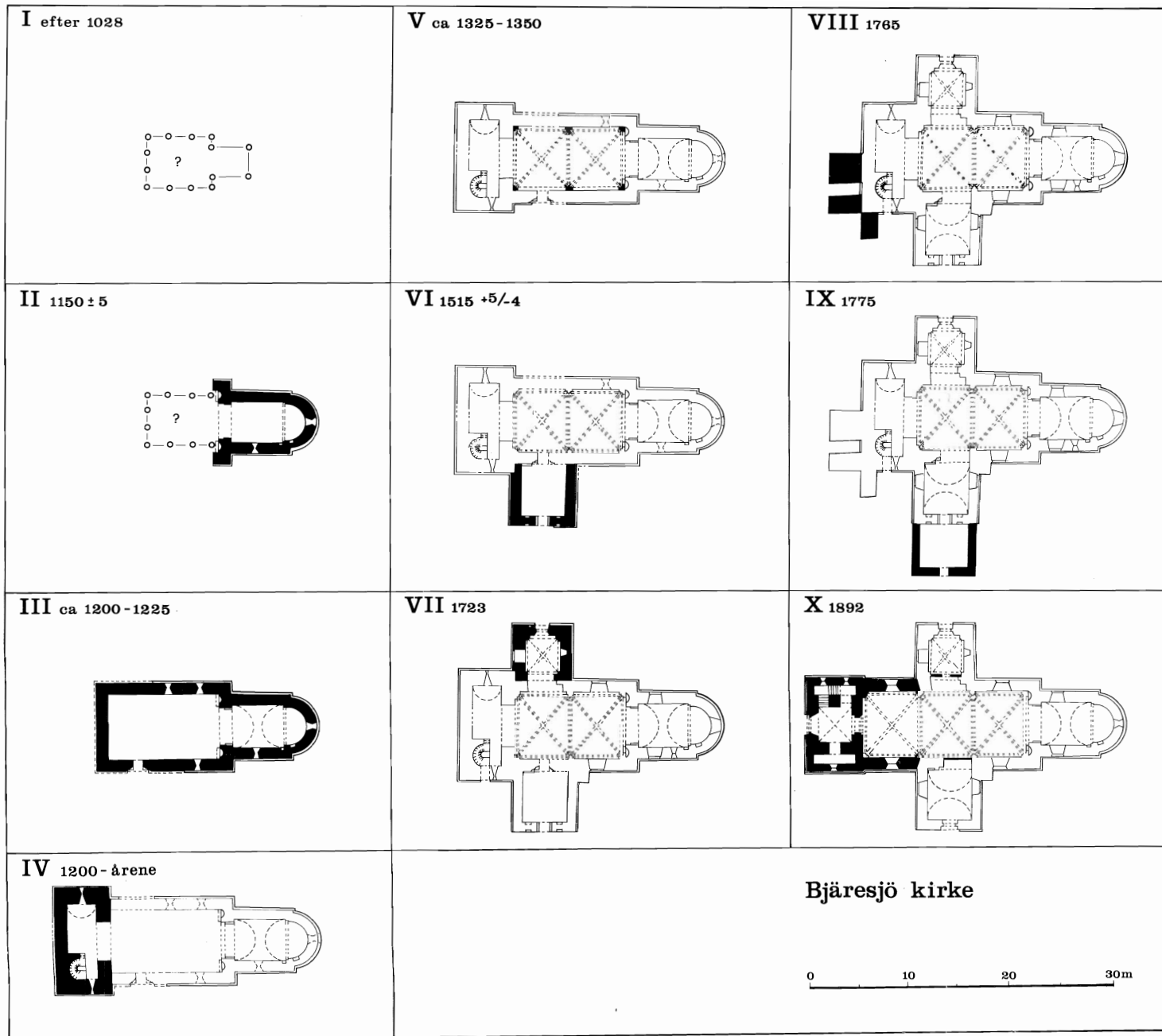
Fig 31. Bjäresjö kirkes planudvikling.
