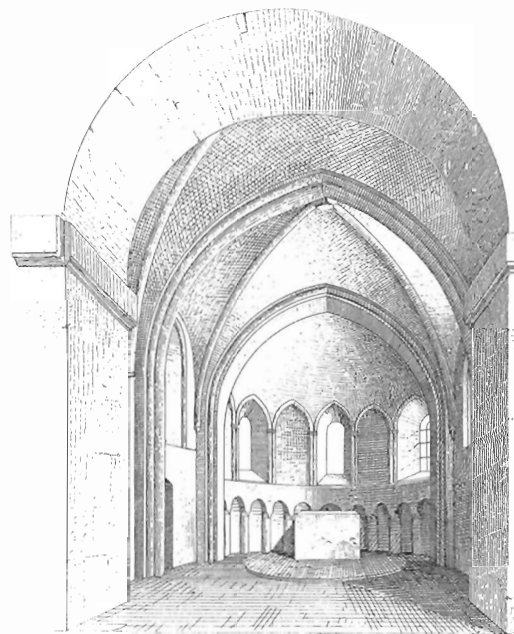
Fig 18. Brøndum kirkes kor og apsis med runde og spidse buer, halvkuppelhvælv og ribbehvælv. Korets tagværk, og dermed hele kirken, er blevet dendrokronologisk dateret til midten af 1240'erne. Skitse af Vilhelm Ahlmann 1891 efter Storck 1903.
