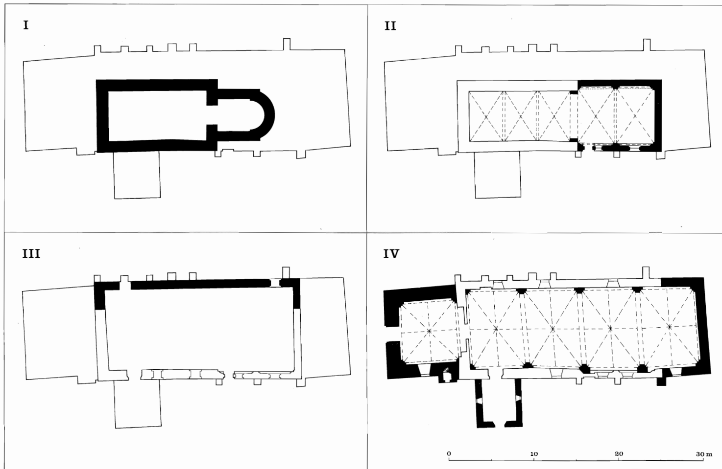
Fig 103. Frørup kirkes udvikling. Valfartskirken blev utvidet og tilbygget flere gange i senmiddelalderen. De komplicerede forandringer er påvist ved en undersøgelse 1974-75. Tegnet efter rekonstruktioner af Morten Aaman Sørensen 1981, Nationalmuseet i København.
