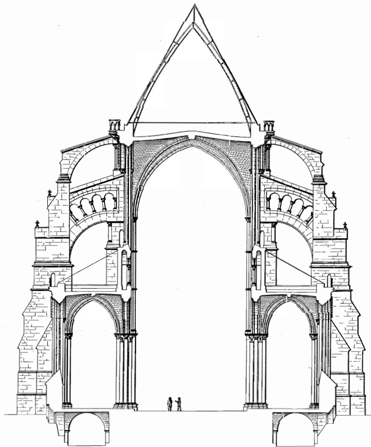
Fig 16. Katedralen i Chartres med gotikkens formale kendetegn, spidsbuen, ribbehvælv og sprængbuen. Tværsnit af skibet opført efter branden 1194. Efter King 1858-68.
