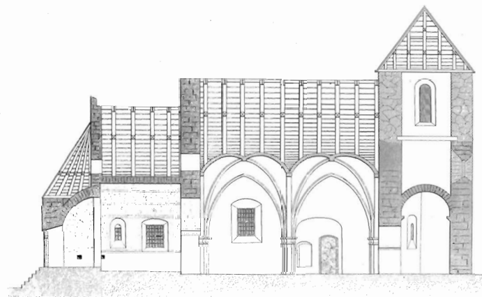
Fig 32. Bjäresjö kirke i længdesnit inden det romanske tårn blev nedbrudt. Efter Mandelgren 1862.
