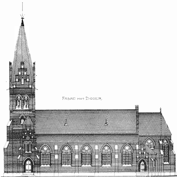
Fig 106. Tygelsjö nye kirke. Tegning af arkitekten A W Lundberg 1901, her retoucheret efter Engman m fl 1991.
