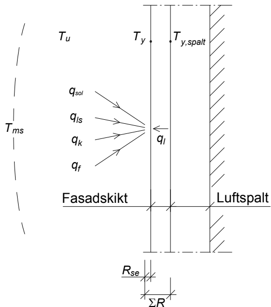
Figur 3-4 Energibalans på utsida av fasadsnittet.
