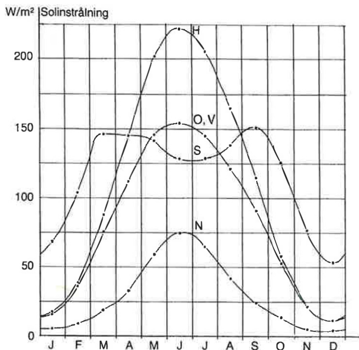
Figur 8-1 Medelsolinstrålning, Malmö (Nevander och Elmarsson, 1994).
