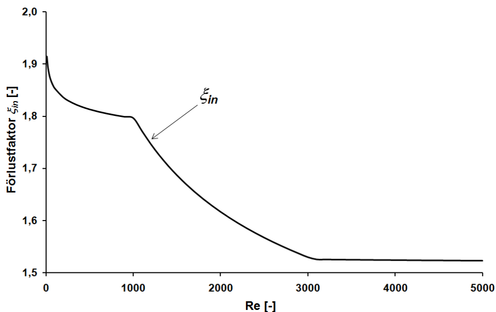
Figur 2-16 Förlustfaktor \xi_{in} (Kronwall, 1980).
