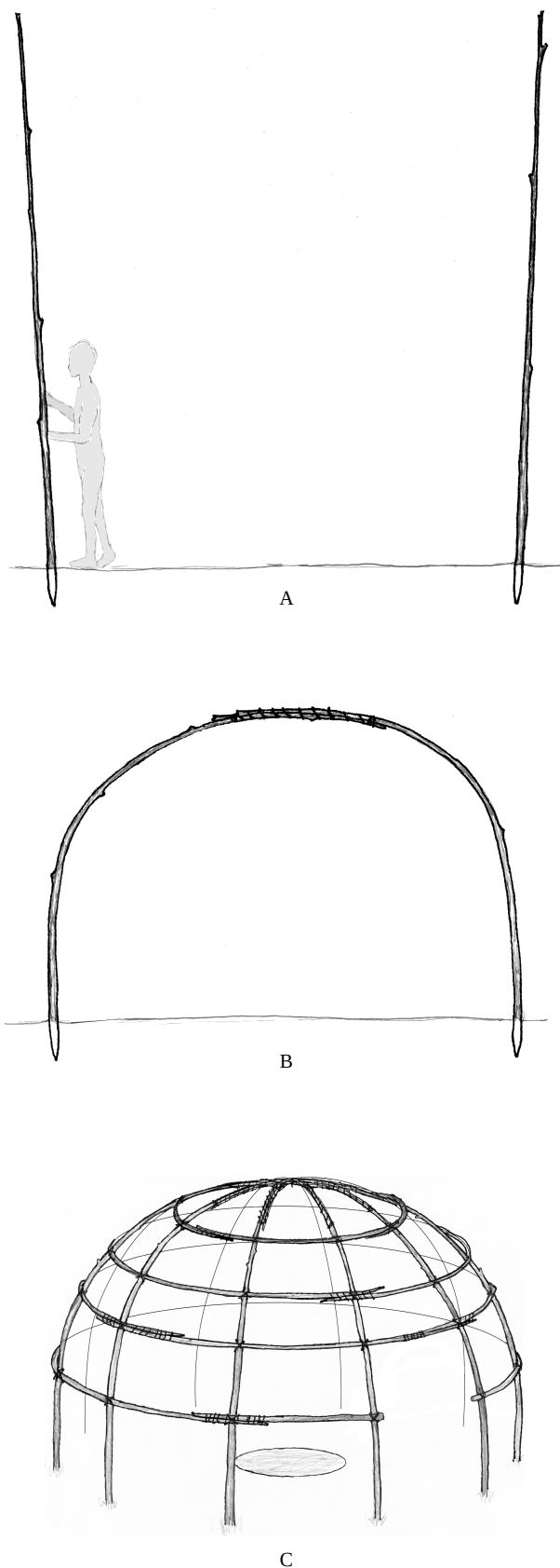
Fig. 48. Principskiss hur man kan ha tillverkat en domformad hydda av långa hasselkäppar: a. den cirkulära eller ovala formen på golvytan bestäms genom att alla käppar placeras ut och körs ner i marken, b. käpparna böjs och binds ihop med motstående käppar, c. tunna tvärgående käppar eller grenar binds ihop med stommen, som slutligen täcks med lämpligt material.
