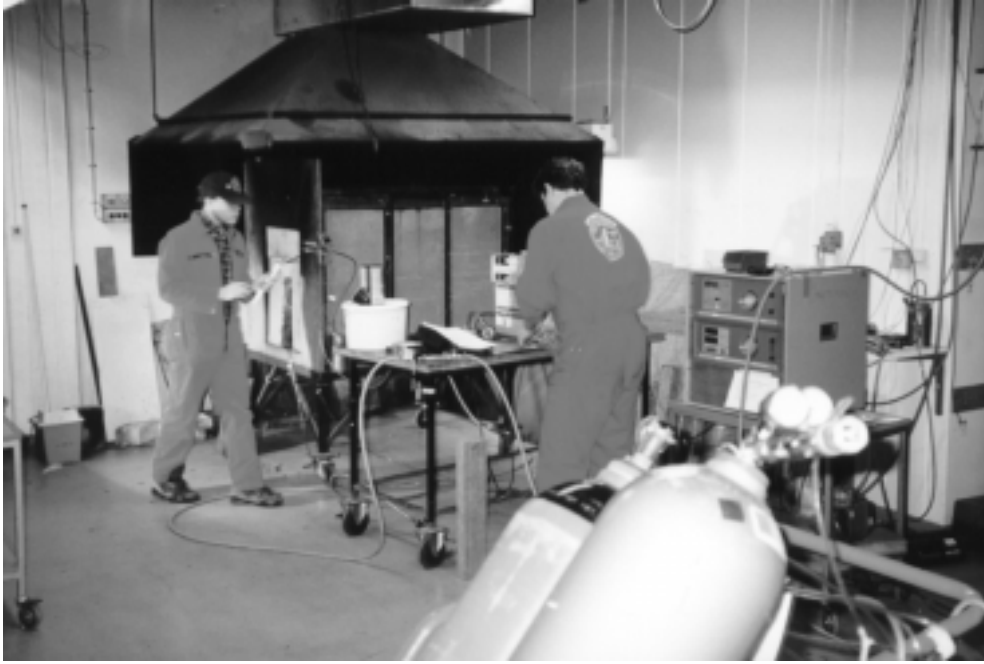
Figur B.1, Försökuppställningen för metanförsöken. Förbränningskammaren ses i bakgrunden under huvan och analysinstrumenten till höger /B.2/.
