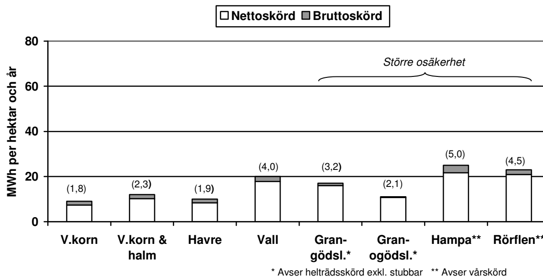
Figur 9.8. Uppskattning av genomsnittlig brutto- respektive nettoenergiskörd per hektar och år för olika energiavslagsgrödor vid odling i Övre Norrland idag. Värdena inom parentes anger hektarskörd i ton torrsubstans per år (relaterade till en vårkornskörd om 2,1 ton). Stubbskörd i granodling medför 10-15 % högre energiskörd.
