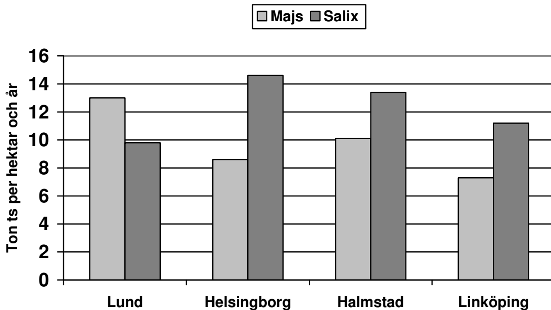
Figur 7.2. Genomsnittlig biologisk skörd (exklusive skördeförluster) av majs och salix i de fyra olika fältförsöken (exklusive etableringsåret för salix) (Törner, 1988).
