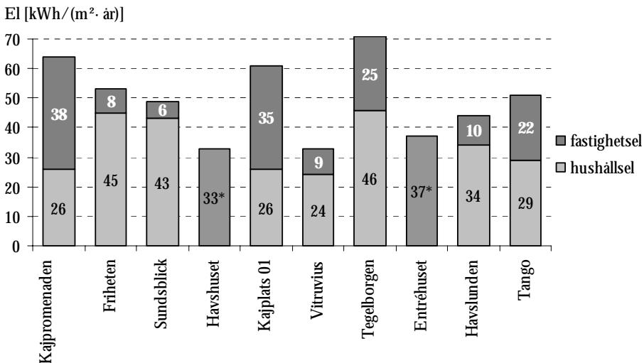
Figur 5:9 Uppmått hushållsel och fastighetsel för de tio fastigheterna. Värderna för Havshuset och Entréhuset inkluderar både hushållsel och fastighetsel.
