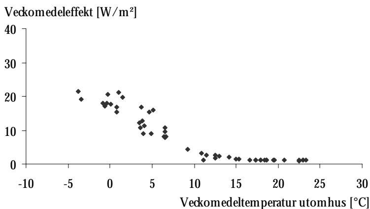
Figur 4:24 Effektsignatur på veckovärden över uppmätt värmeeffekt för Kajplats 01, plottad mot motsvarande uppmätt utetemperatur på Bo01-området.
