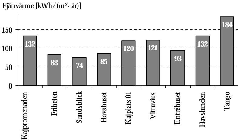
Figur 5:2 Uppmätt, normaliserad fjärrvärmeanvändning där arean för garage är borträknad för de fastigheter som har inkluderat garaget i sina beräkningar.
