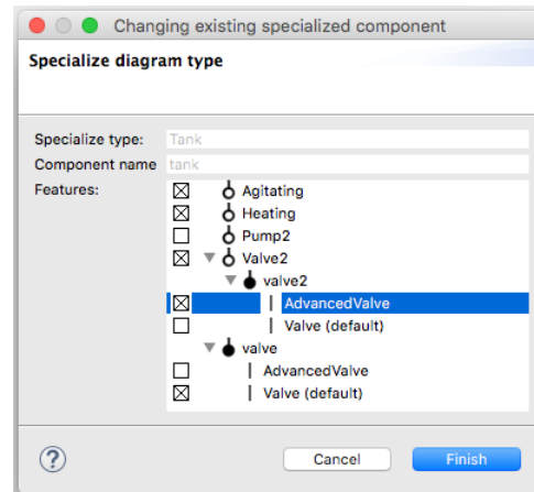
Figur 2. Utvecklaren skapar styrprogram för en tank och kan välja vilken funktionalitet tanken ska ha.
