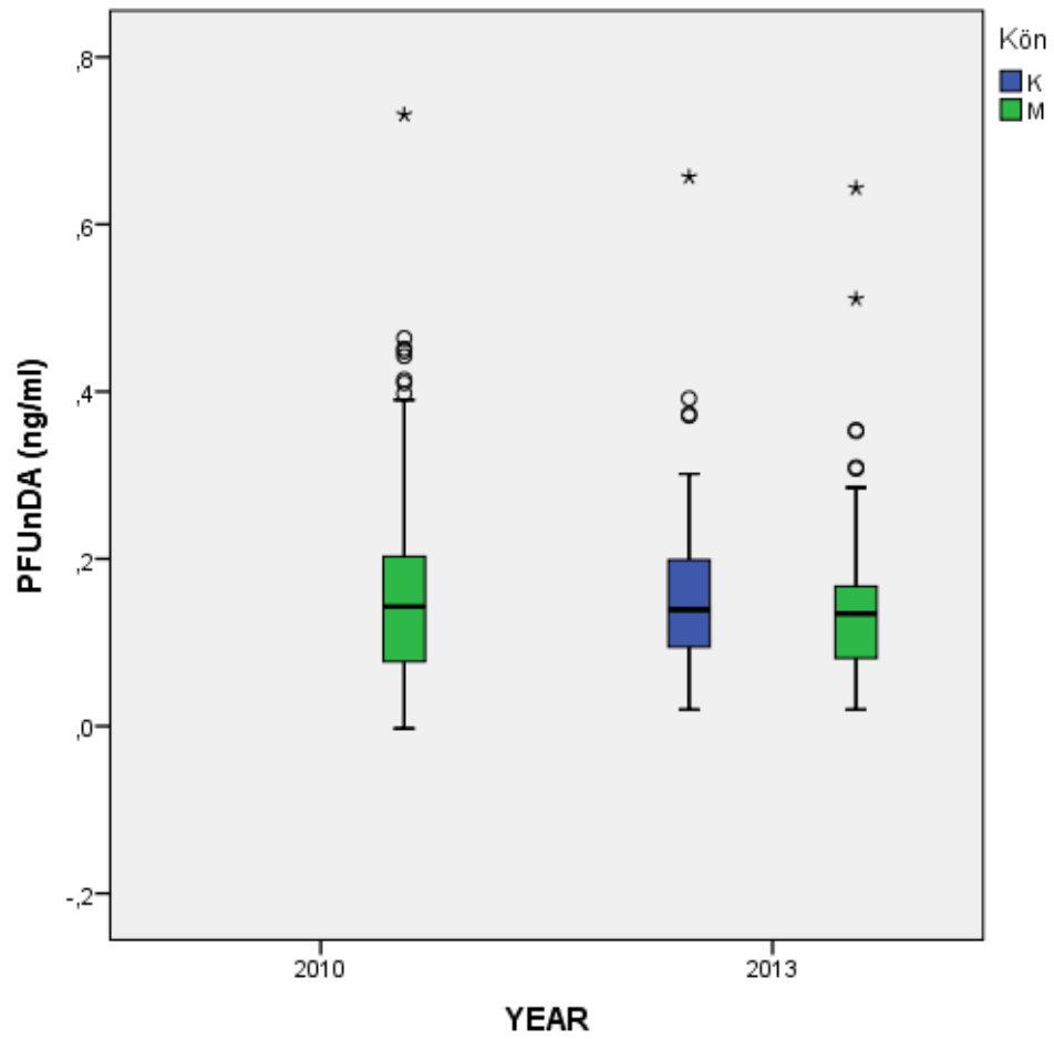
Figur 6: Box-plott av halterna av PFUnDA från män år 2010 samt män och kvinnor år 2013.
