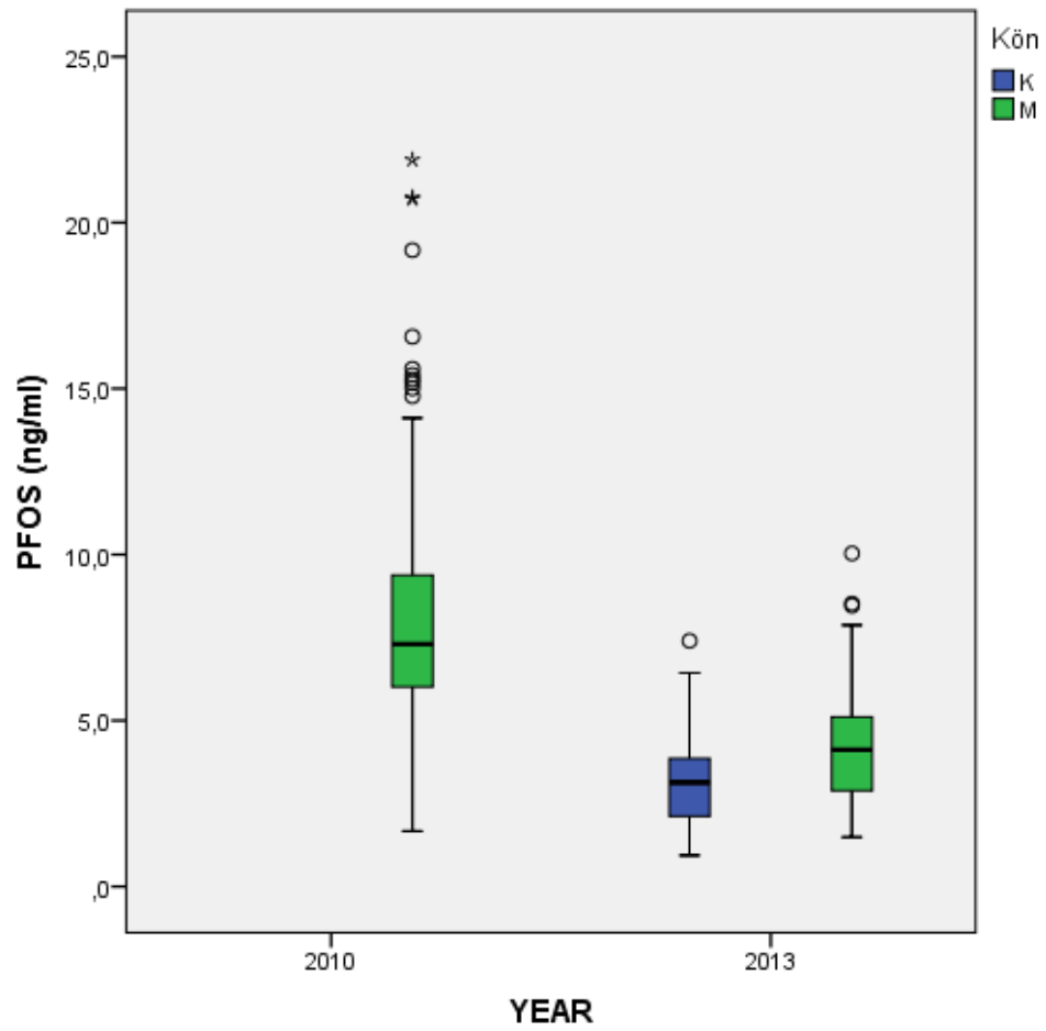
Figur 2: Box-plott av halterna av PFOS från män år 2010 samt män och kvinnor år 2013.
