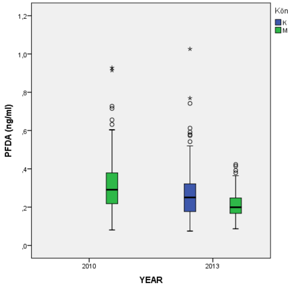
Figur 5: Box-plott av halterna av PFDA från män år 2010 samt män och kvinnor år 2013.
