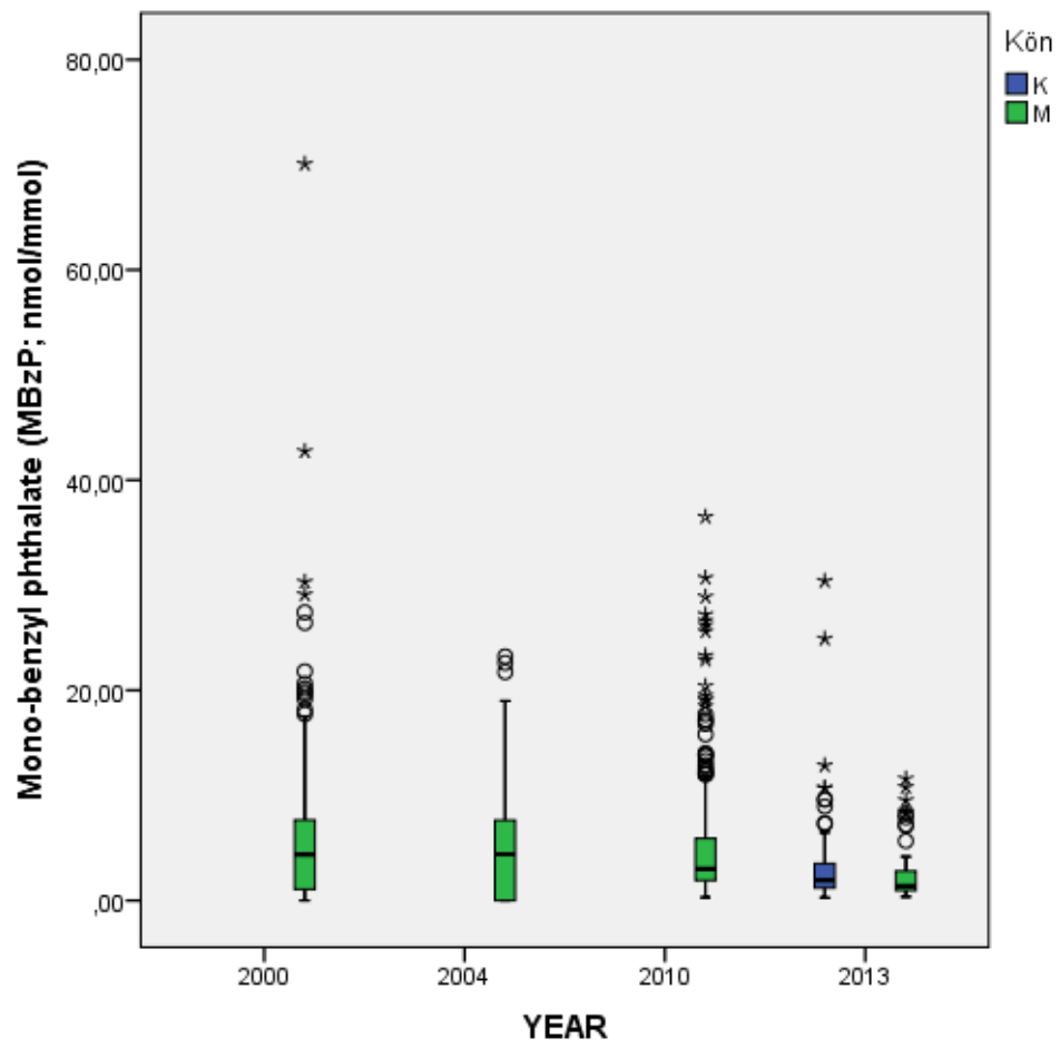
Figur 9: Box-plott av halterna av MBzP från män år 2000, 2004, 2010 och 2013 samt kvinnor år 2013.
