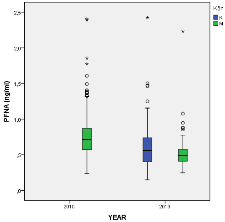
Figur 4: Box-plott av halterna av PFNA från män år 2010 samt män och kvinnor år 2013.
