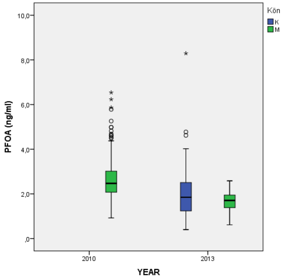
Figur 3: Box-plott av halterna av PFOA från män år 2010 samt män och kvinnor år 2013.
