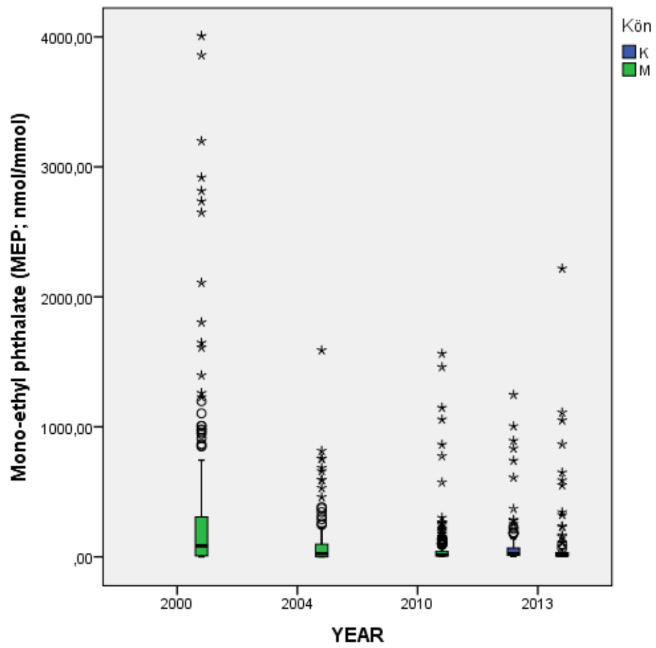
Figur 7: Box-plott av halterna av MEP från män år 2000, 2004, 2010 och 2013 samt kvinnor år 2013.
