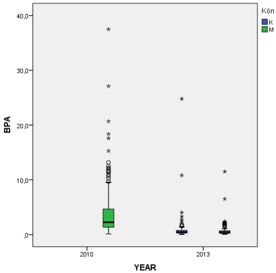
Figur 11: Box-plott av halterna av bisfenol A (BPA) från män år 2010 och 2013 samt kvinnor år 2013.
