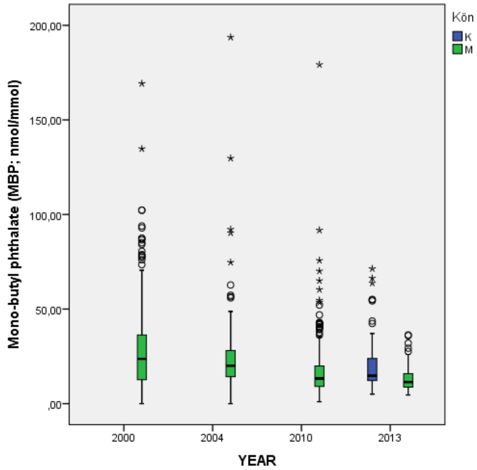
Figur 8: Box-plott av halterna av MBP från män år 2000, 2004, 2010 och 2013 samt kvinnor år 2013.
