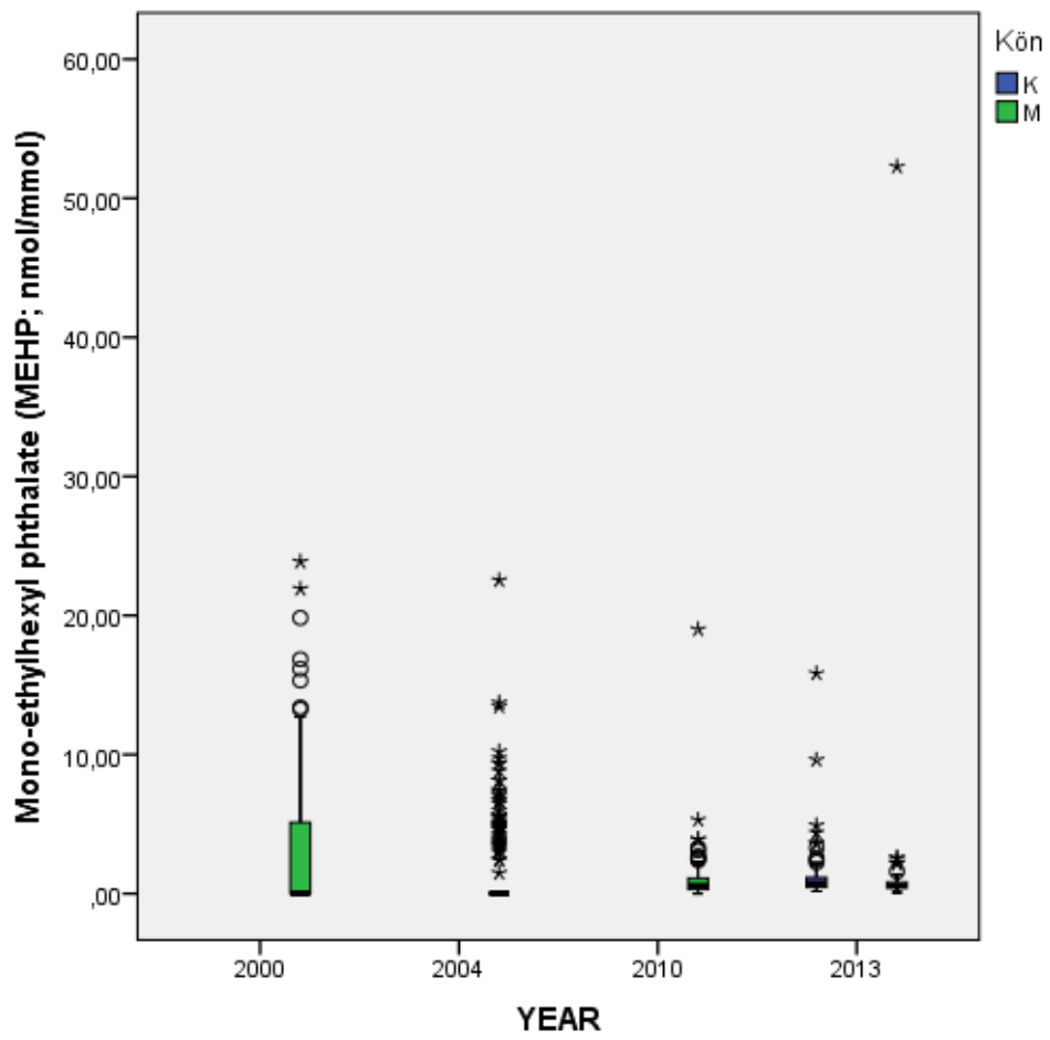
Figur 10: Box-plott av halterna av MEHP från män år 2000, 2004, 2010 och 2013 samt kvinnor år 2013.
