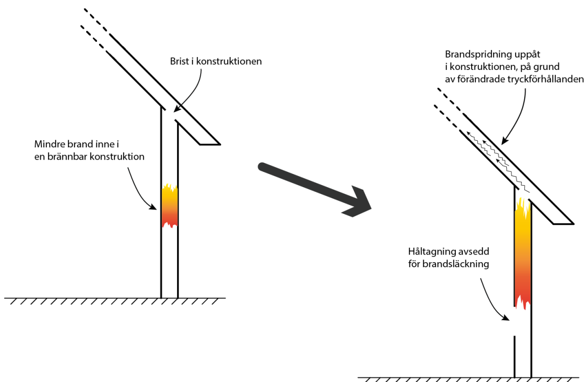
Figur 16; Enkelt exempel på skorstenseffektens verkan i en brännbar konstruktion.
