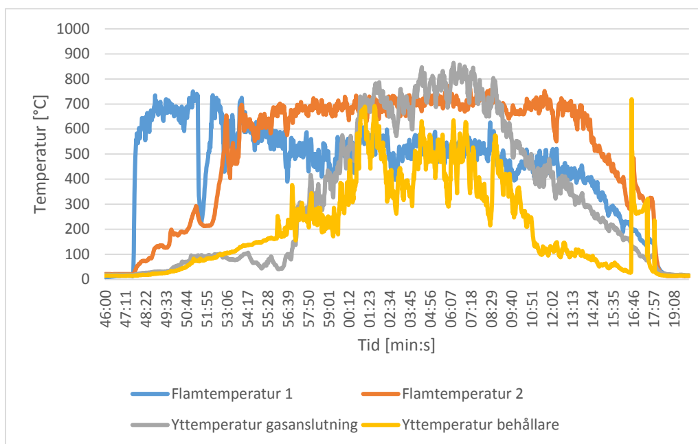
Figur 37. Temperaturer under brandprovning 1 med gasolbehållare
