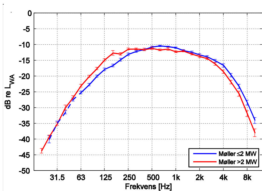
Figur 4. Normerede A-vægtede lydeffektniveauer i 1/3-oktavbånd. Middelværdier for to grupper af møller: \square 2 MW og \square > 2 MW. Lodrette streger angiver \pm 1 standard error of mean (s.e.m.).
