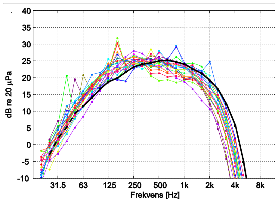
Figur 6. A-vægtet lydtrykniveau i 1/3-oktavbånd ved den afstand fra hver enkelt mølle, hvor det totale A-vægtede lydtrykniveau er 35 dB (se Tabel 1). Farvekode for møller som i Figur 5.
