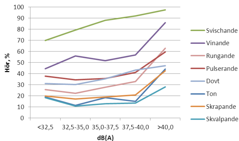
Figur 2. Andelen som hörde de olika ljudkaraktärerna av de svarande som uppgett att de hörde ljud från vindkraftverk i de svenska studierna ( n = 520 ). Andelen som hörde vindkraftverken var lägre bland de som inte kunde se några vindkraftverk från sin bostad än bland de som såg ett eller flera verk, även när de beräknade ljudnivåerna var lika. De som inte såg vindkraftverken var troligen exponerade för lägre ljudnivåer än de beräknade, kanske för att en byggnad skymde sikten och därmed också dämpade ljudet. Men det kan också vara så att avsaknaden av visuellt intryck gjorde dem mindre uppmärksamma på ljudet. När två sinnen stimuleras samtidigt så ökar den totala uppmärksamheten (multimodal effekt) så att, i det här fallet, ljud som annars inte skulle ha gett någon respons uppfattas.
