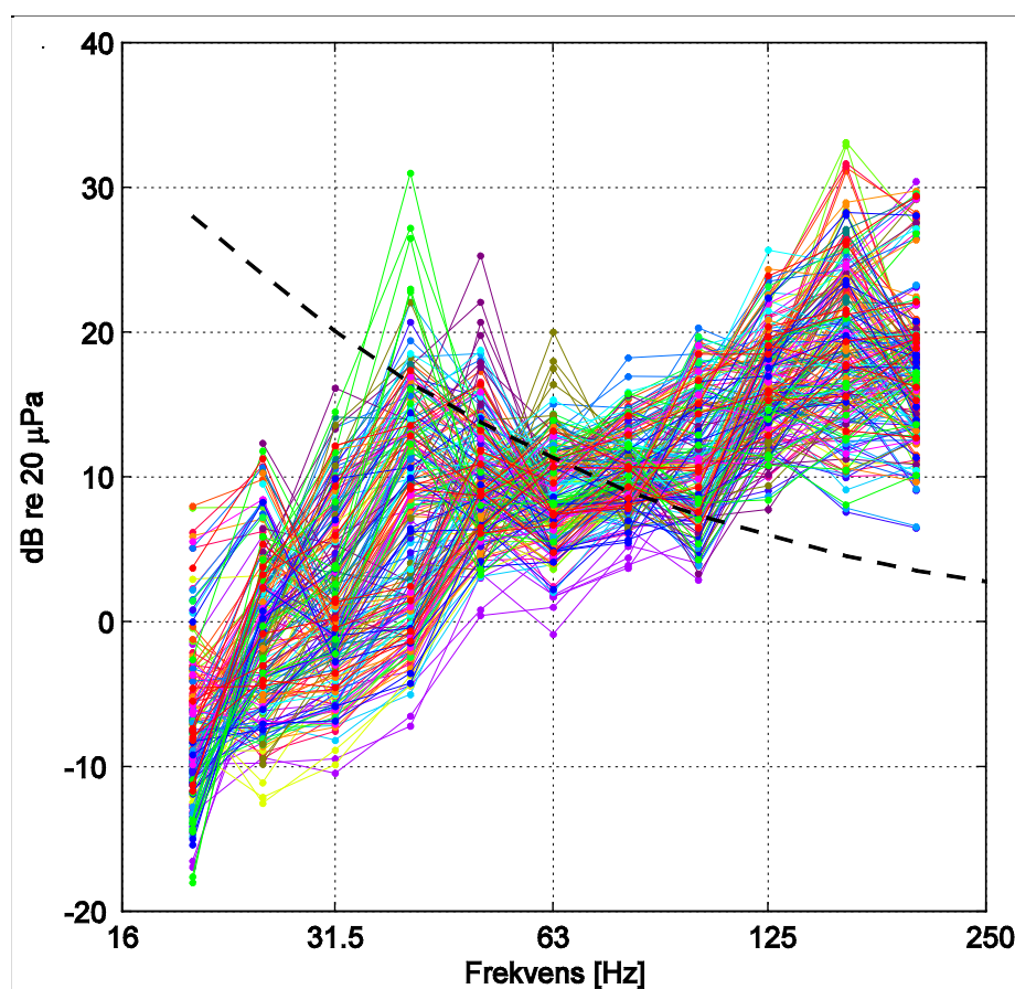
Figur 9. Indendørs A-vægtede lydtrykniveauer for 1/3-oktavnånd i den afstand fra en m llepark, hvor det totale A-v gtede lydtrykniveau udend rs er 44 dB (se Tabel 2). 207 kombinationer af 23 store m ller og 9 rum. Stiplet linje er h ret rsklen i henhold til ISO 389-7. Farverne angiver m llen, farvekode som i Figur 5.
