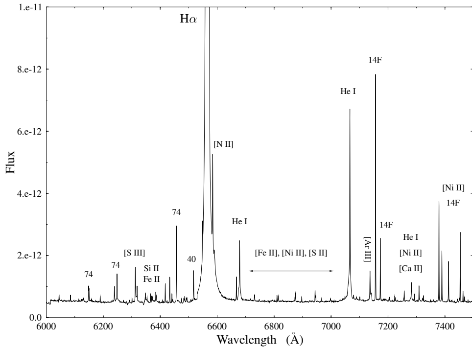
Fig. A.8. The 6000–7500 Å spectrum.
