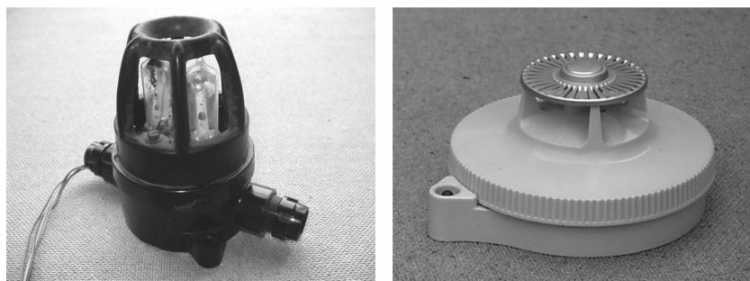
Figur 3.12 Två värmedetektorer av äldre modell
