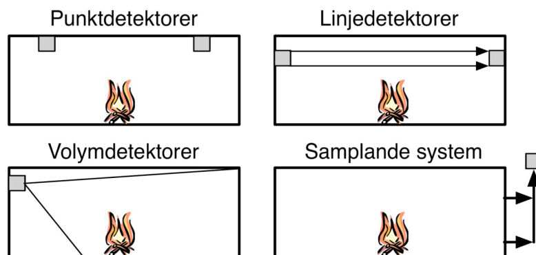
Figur 2.2 Principerna för punktdetektorer, linjedetektorer, volymdetektorer och samplande system. Detektorerna är grå kvadrater i bilden.
