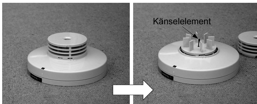
Figur 3.11 Värmedetektor som sönderdelas.
