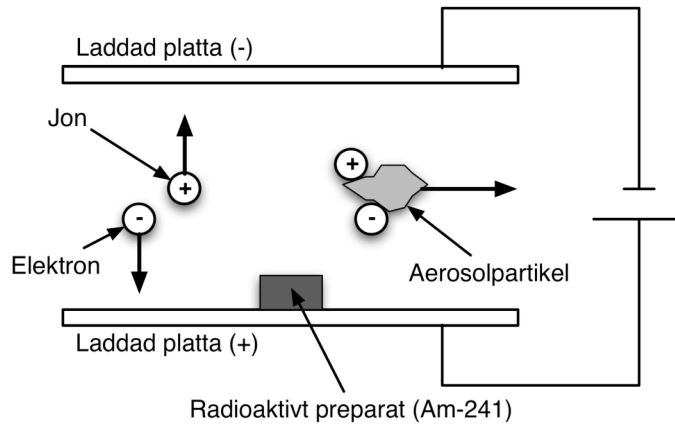
Figur 2.4 En joniserande rökdetektors funktion
