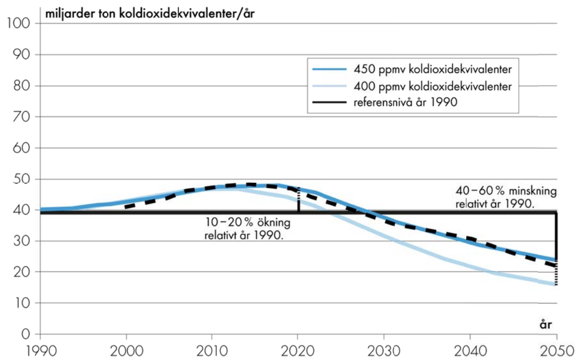
Figur 4.5.2. Jämförelse mellan en utsläppsbana genererad i MiMiC (streckad linje) och de i MVB-SOU (2007) analyserade utsläppsbanorna. Notera att banorna visas endast fram till år 2050.
