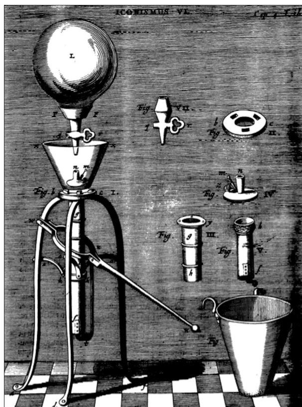
Fig. 7. von Guericks luftpump av den tredje förbättrade typen som ingår i Lunds universitets instrumentsamling. Notera spannen till höger som ska vattenfyllas och hängas på trefoten under cylindern för att motverka läckage. Ur Otto von Guericke, Experimenta Nova Magdeburgica (1672).
