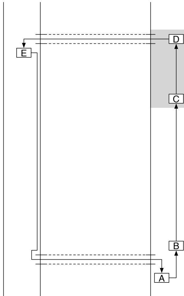
Figur 11. Schematisk beskrivning av försöksområdet. Höger del av figuren illustrerar Norrtullstunneln och vänster del Gärdéstunneln. Gråmarkerad yta illustrerar den rökfyllda delen av försöksområdet.
