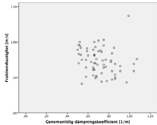
Figur 31. Genomsnittlig fraktionshastighet i rök som funktion av dämpningskoefficienten. Utdata från SPSS.
