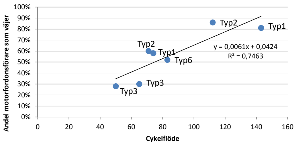
Figur 37: Samma som figur 36 men här redovisas diagrammet i form av de olika typerna av cykelöverfarter/passager och deras samband med cykelflöde och andel motorfordonsförare som väjer. En rät linje anpassas till punkterna.
