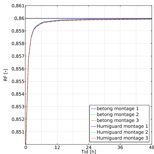
Figur 20. Beräknad fuktighet i HumiGuard-sensor och betong efter första, andra och tredje montaget i ett och samma borrhål.
