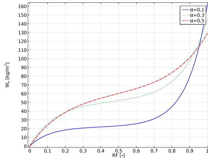
Figur 7. Sorptionsisoterm för betong vct 0,38 med olika \alpha=0,1 ; 0,3 och 0,5
