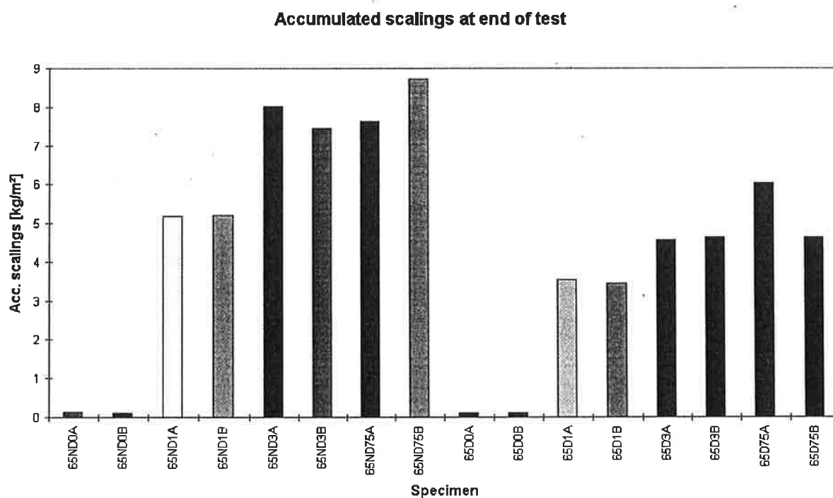
Figur 6: Slutlig avskalning för huvudserie 2, vct 0.65 (9 cykler)
