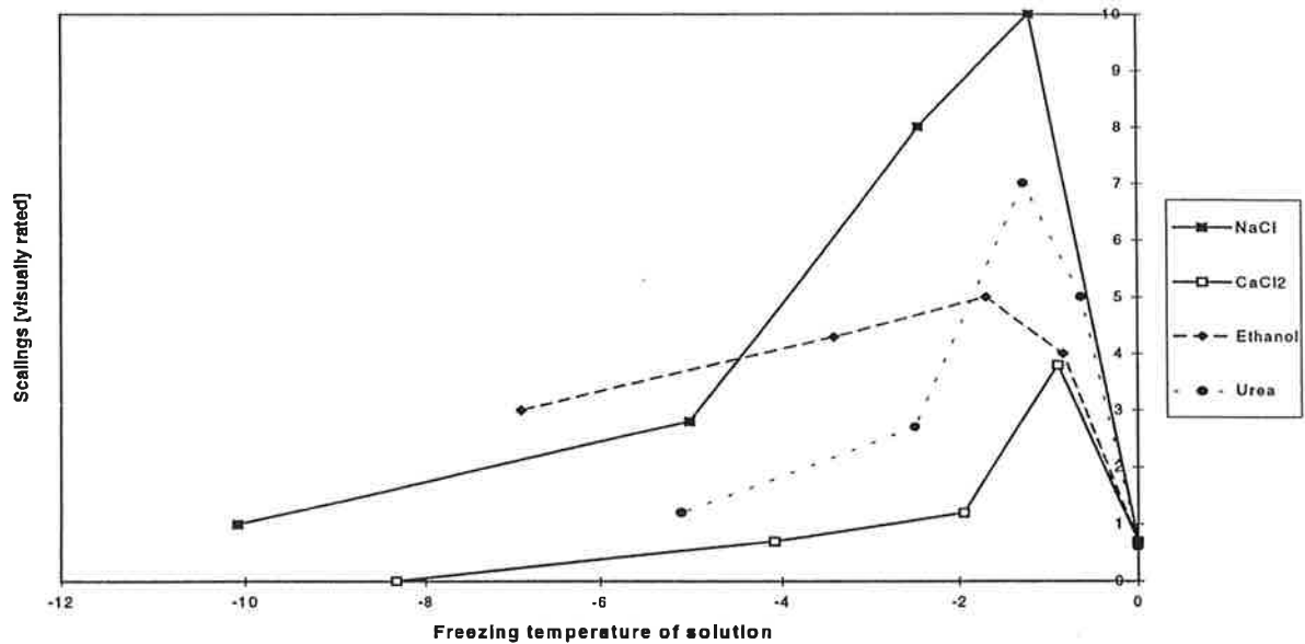
Figur 1: Bearbetning av resultat från Verbeck och Klieger [3]. Visuell bedömning av ytskadorna mot fryspunktssänkningen för det aktuella avisningsmedlet.
