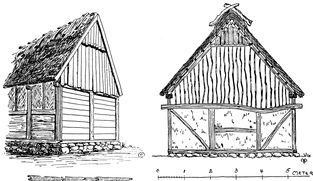
Exempel på Mårten Sjöbecks ritningar. Typisk gavelkonstruktion från Vitteröd, Munkarps s:n, Frosta h:d, resp. Besshus, Ekeby s:n, Luggude h:d. Ur Hälsingborgs Museums Årsskrift 1928.
