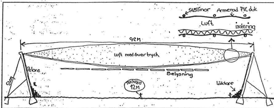
Figur 4.1. Takkonstruktion med ställinor och armerad PVC-duk för stora spännvidder [13].
