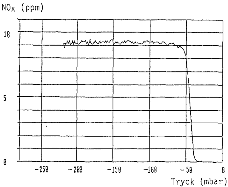
Figur 2.8c Tryckoberoende mätsignal
