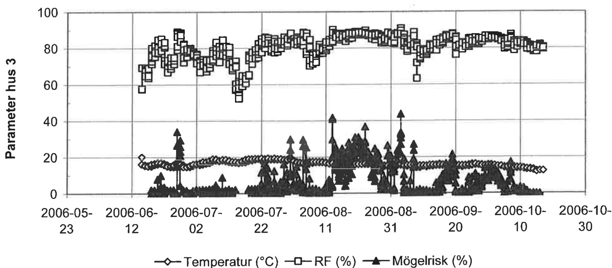
Figur 3 - Temperatur, RF och risk för mögelpåväxt på obehandlat trä (gran) 2005-2006.
