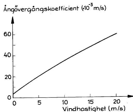
FIG. 7:21. Samband mellan ångövergångskoefficient och vindhastighet enligt van der Held (1941).
