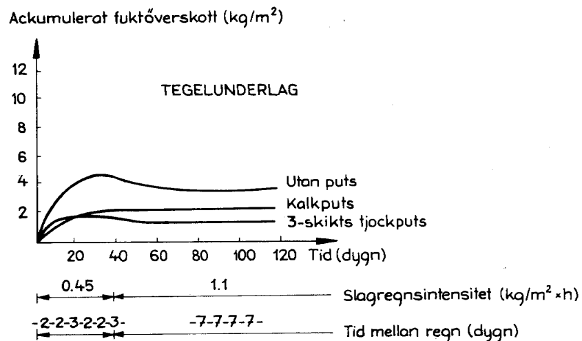
FIG. 7:28. Medelfukthinnehållets förändring vid cykliskt återkommande slagregn. Regnets varaktighet har alltid varit 3 \frac{1}{4} h. Mean moisture content at cyclic driving rains with duration 3 \frac{1}{4} h.
