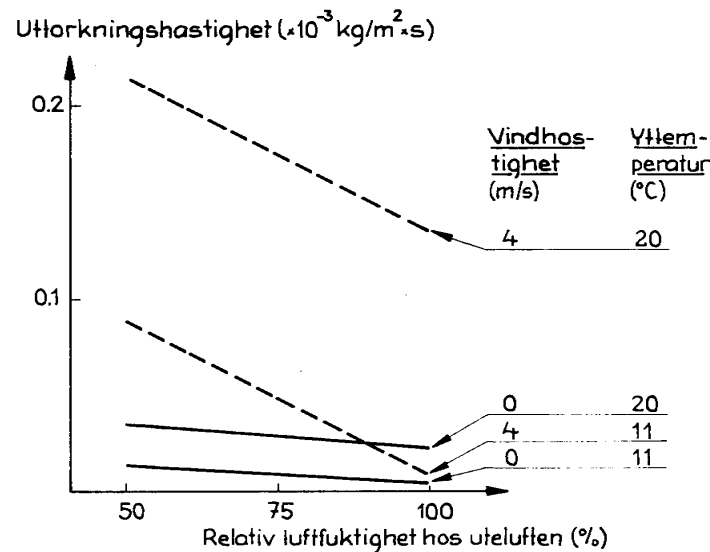
FIG. 7:22. Uttorkningshastighetens beroende av lufthastighet och ytttemperatur vid avdunstning från ytan. Lufttemperatur 10^{\circ}\text{C} .
