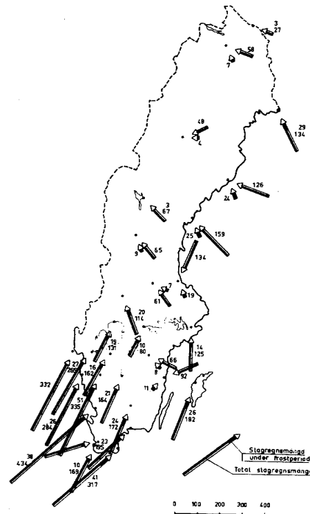
FIG. 7:9. Årlig slagregnmängd ( \text{kg/m}^2 ) som träffar fasader vända mot den för slagregn farligaste riktningen för respektive ord. (Varnbo, 1966). Annual amount of driving rain ( \text{kg/m}^2 ) against facades in "the most dangerous" direction.
