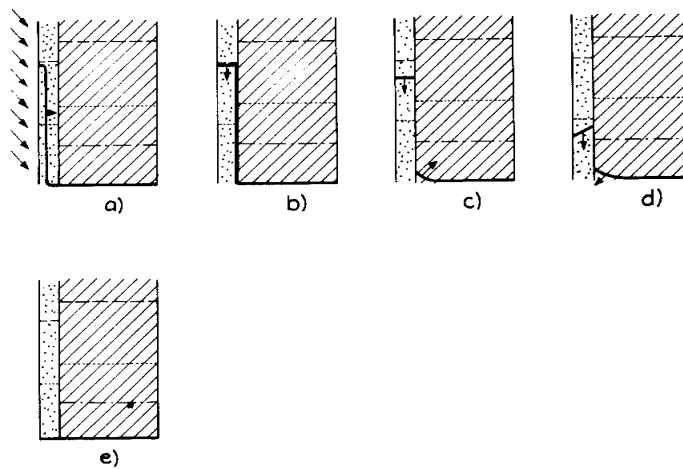
FIG. 7:25. Fuktförlopp under och efter ett litet slagregn.
