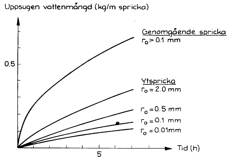
FIG. 7:17. Beräknad uppsugen vattenmängd i gasbetong med tätt ytskikt och olika sprickor med bredden 2r_o .
