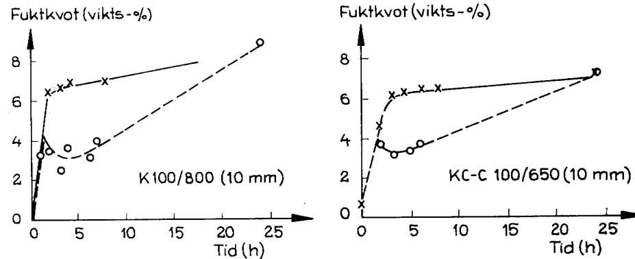
FIG. 7:16. Medelfuktkvot i putsen som funktion av tiden under slagregn med intensiteten 0.45 \text{ kg/m}^2 \cdot \text{h} .
