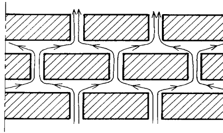
FIG. 7:32. Kapillärsugning i fogar till ett murverk med stenar som ej suger vatten.
