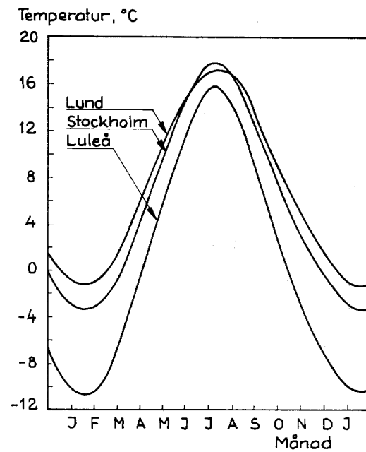
FIG. 7:3. Dygnsmideltemperaturens årsvariation för Lund, Stockholm och Luleå baserad på månadsmedeltemperaturer. 1931-1960. (Sandberg, 1973). Annual variation of daily mean temperature in some Swedish places.
