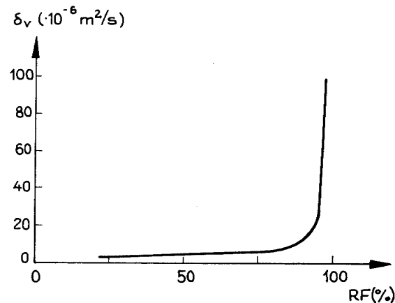
FIG. 6:5. ÄnggenomslÄpplighetskoefficienten som funktion av RF fÖr gasbetong enligt delrapport IV.
