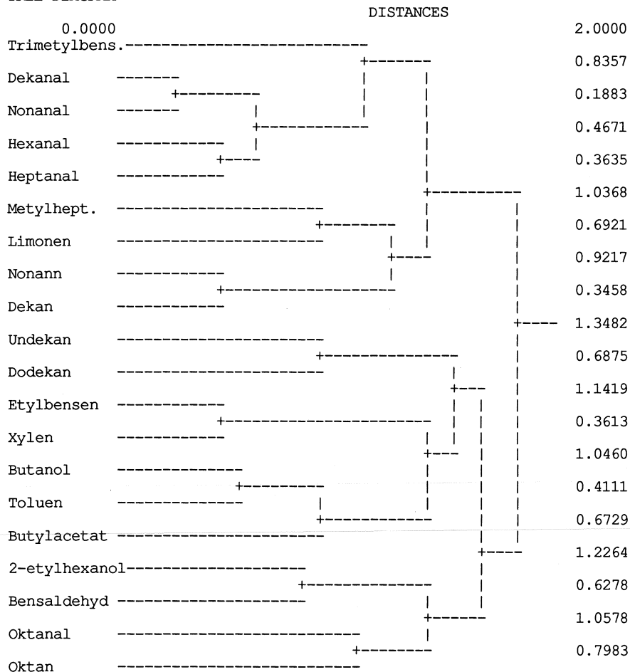
Figur 7.16 Hierarchical Cluster analys (Distance metric; 1-Pearson coefficient complete linkage method) av 20 enskilda VOC-ämnena i inomhusluften som förekommer i mer än 10 % av de 66 undersökta lägenheterna. Av analysen framgår att det fanns ett antal kemikaliegrupper där enskilda VOC-ämnena korrelerade internt med avseende på koncentrationen. En grupp utgjordes av 2-etylhexanol och bensaldehyd samt oktanal och oktan. Det fanns även en grupp med aldehyderna dekanal, nonanal, hexanal och heptanal. En grupp bestod av metylheptanon, limonen, nonan och dekan och en av etylbensen, xylen, butanol, toluen och butylacetat.
