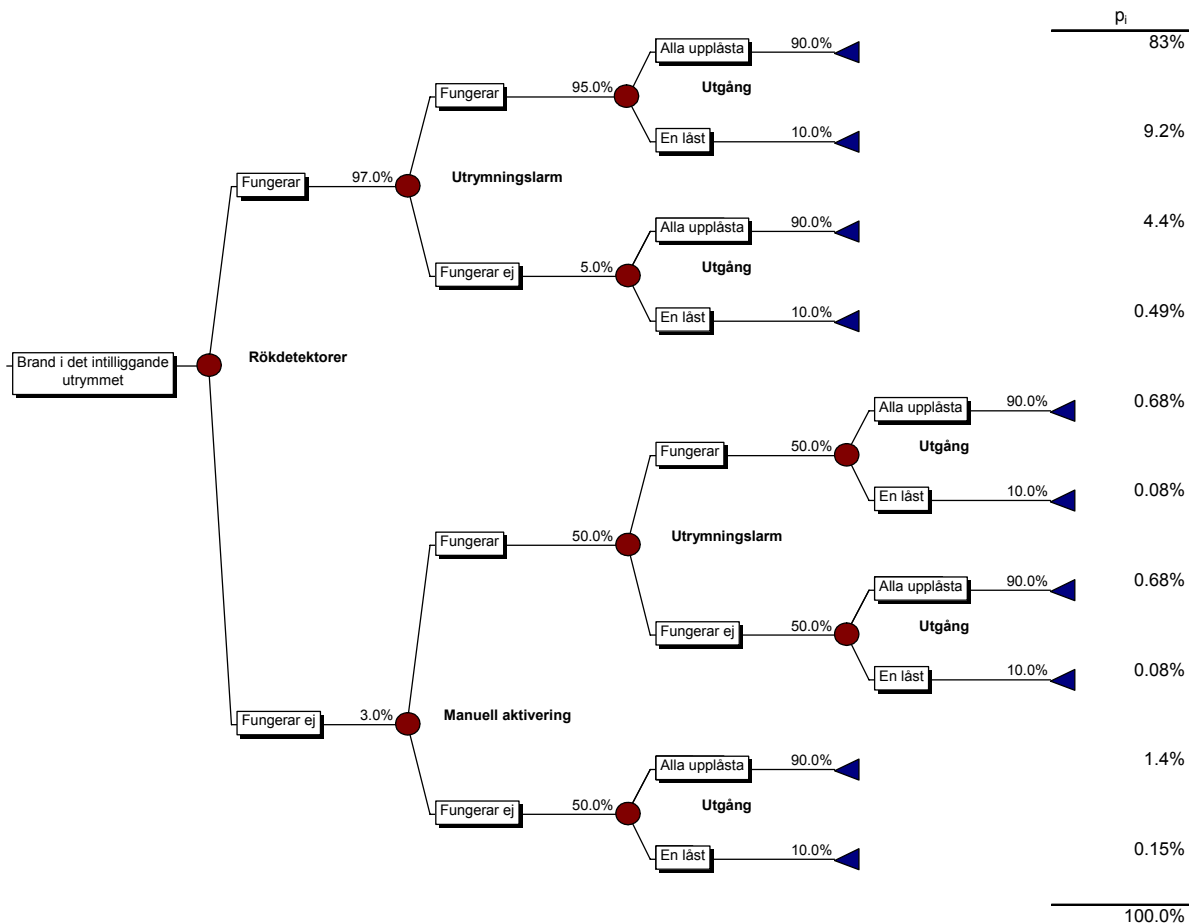
Figur 12. Händelsetråd för brand som startar i ett intilliggande utrymme till samlingslokalen.
