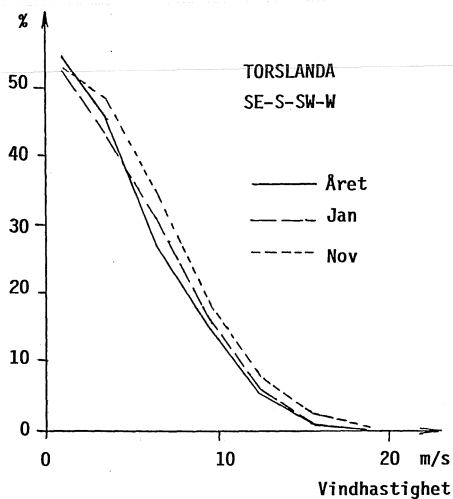
Figur D2. Fördelningskurva för vindhastigheter. Torshanda SE-S-SW-W.
