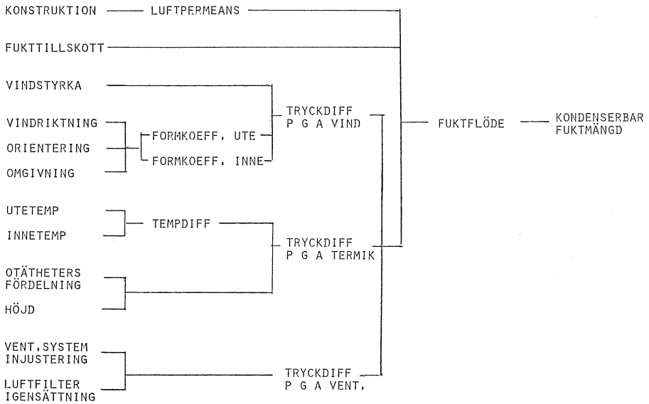
Figur 3.9. Händelseträ för fuktkonvektion genom en byggnadsdel. FT-ventilation.
