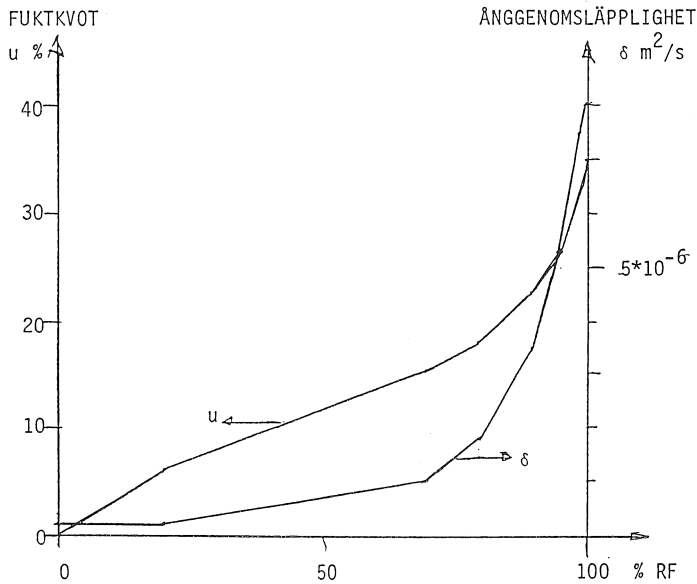
Figur 3.4. Sorptionskurva och ånggenomsläpplighet \delta för trä \perp fibrerna.
