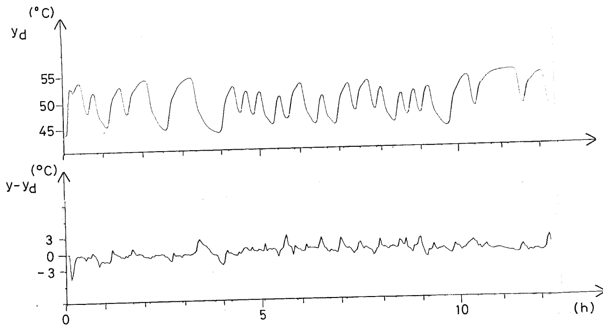
Fig. II:9 - y -deterministisk för 3:e ordn. modell samt skillnaden mellan verklig utsignal och y -deterministisk för 3:e ordningen som funktion av tiden för fall I (hel amplitud).
