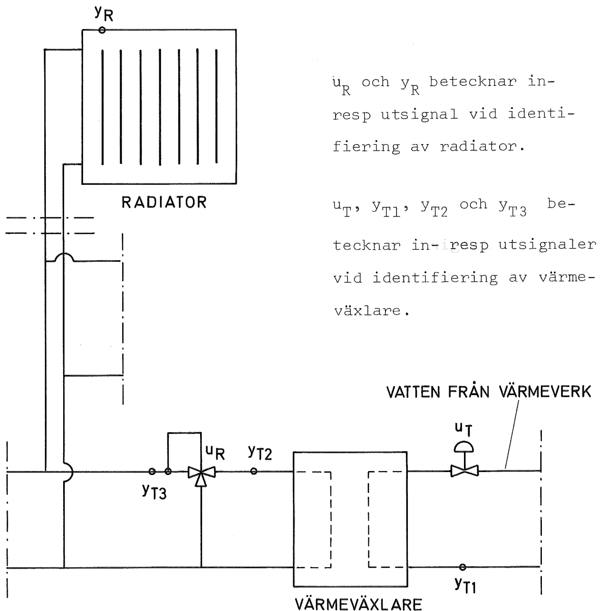
Fig. I:1 Schematisk bild av de identifierade systemen.
