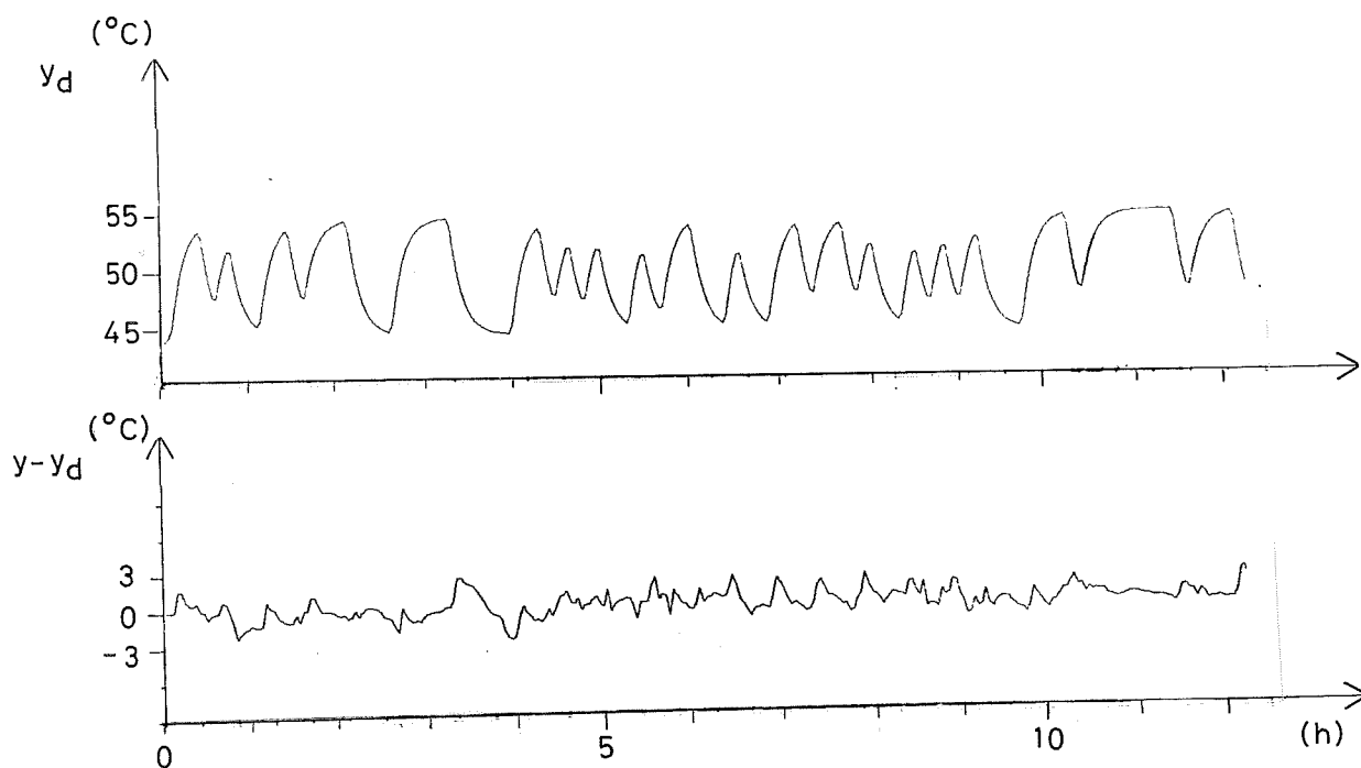
Fig. II:8 - Simulerad utsignal utan störning, y -deterministisk ( y_d ) för 2:a ordningens modell samt skillnaden mellan verklig utsignal och y -deterministisk för 2:a ordningen som funktion av tiden för fall I (hel amplitud).
