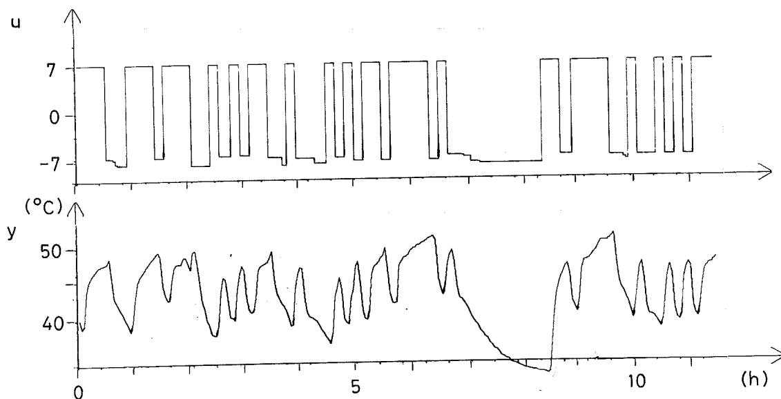
Fig. II:12 - Insignalen ( u ) och utsignalen ( y ) som funktion av tiden för fall II (halv amplitud).
