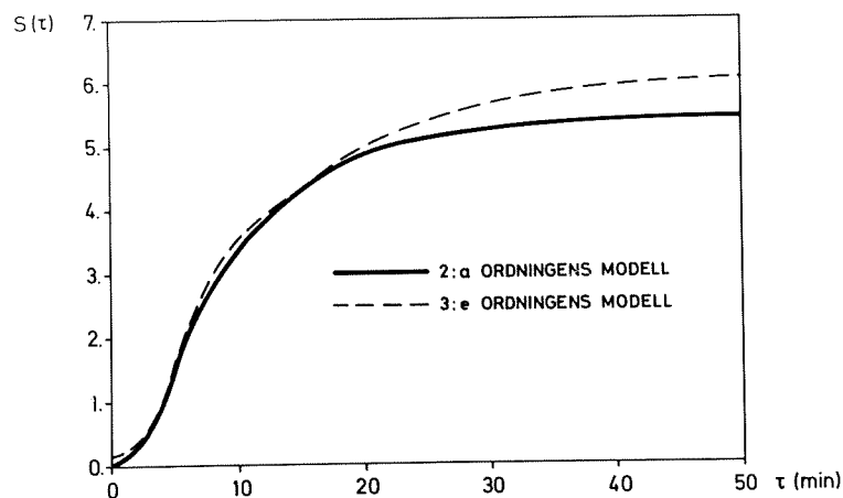
Fig. II:6 - Stegsvaret ( S(\tau) ) för 2:a och 3:e ordn. modell. Fall I (hel amplitud).
