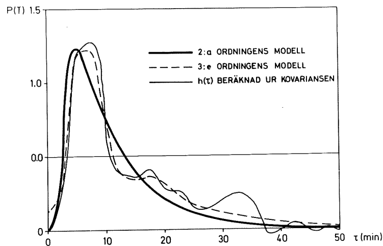
Fig. II:5 - Impulssvaret ( P(\tau) ) för 2:a och 3:e ordn. modell samt viktfunktionerna ( h(\tau) ), beräknade ur kovarianskurvorna. Fall I (hel amplitud).
