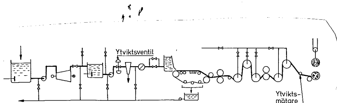
Fig. 8.1 - Förenklad bild av en pappersmaskin.
