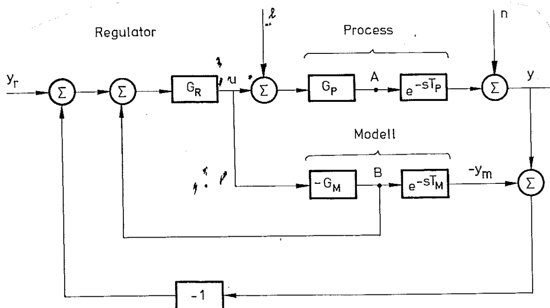
Fig. 8.6 - Blockschemat för process som regleras med Smith's prediktor. Blockschemat för regulatorn representerar ekvationen (8.5).
