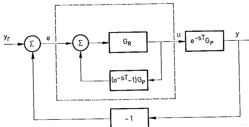
Fig. 8.4 - Blockschema för Smith's prediktor för dödtidskompensering.
