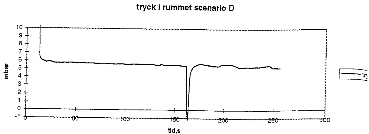
Figur 37. Tryck i rummet scenario D.
