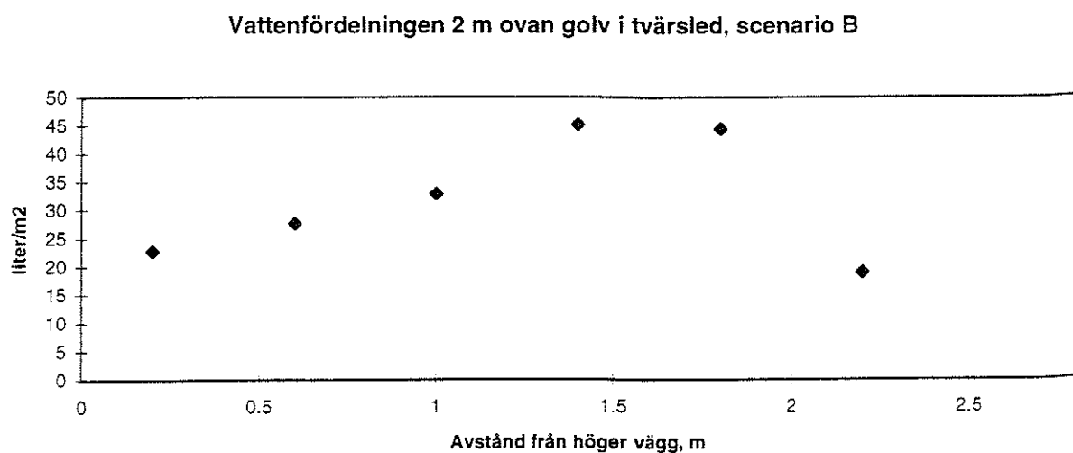
Figur 54. Vattenfördelning i tvärsled 2 m ovan golv.
