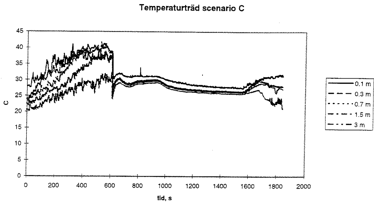
Figur 70. Temperaturträd scenario C.
