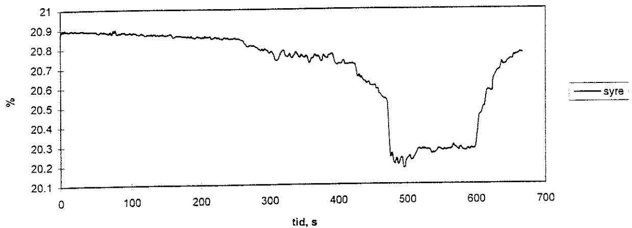
Figur 113. Syrekoncentrationen försök 4.
