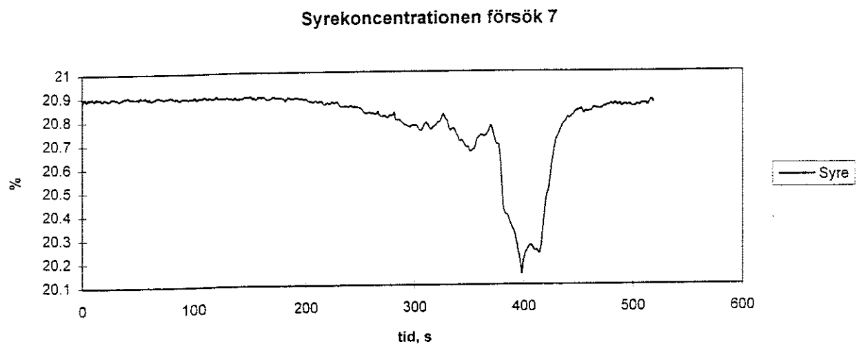
Figur 142. Syrekoncentrationen i rummet försök 7.
