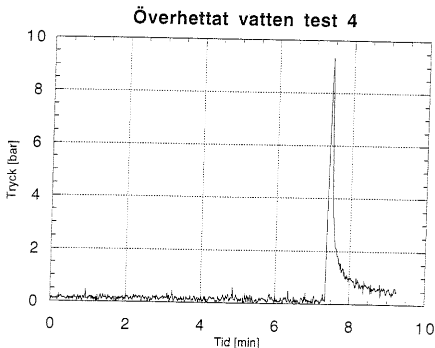
Figur 106. Trycket i munstycket försök 4.
