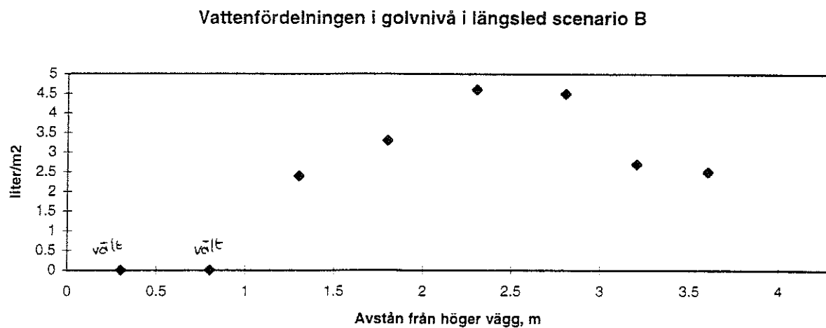
Figur 14. Vattenfördelning längsled på golvet
