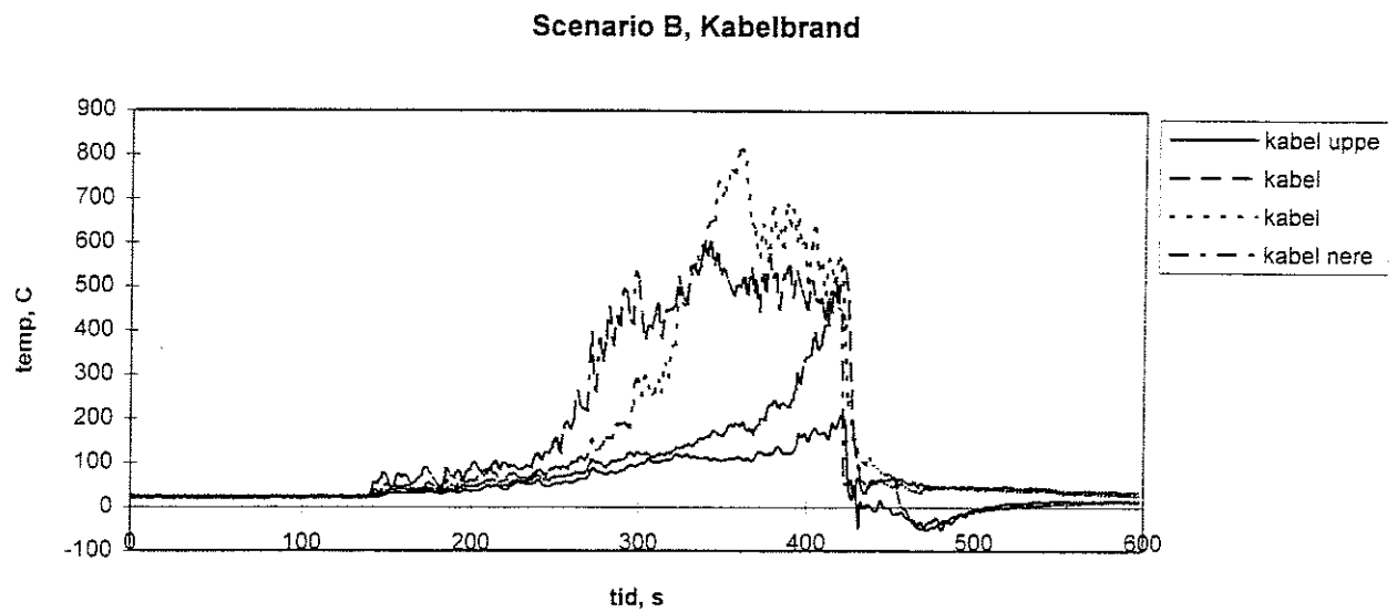
Figur 18 Temperatur vid kabelbranden.
