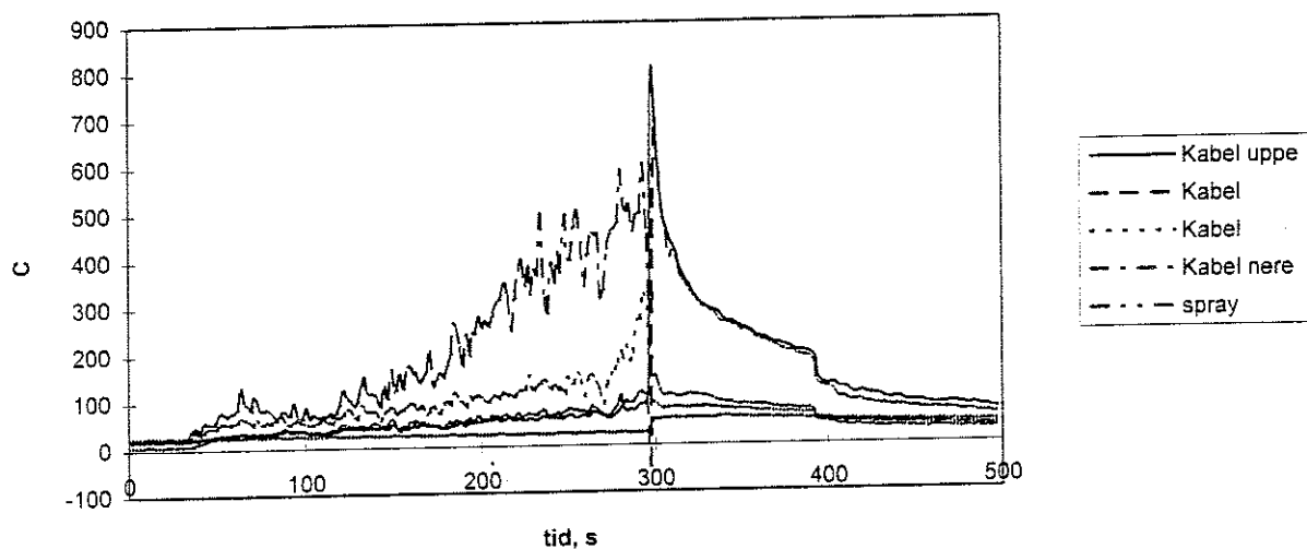
Figur 127. Kabelbranden försök 6.
