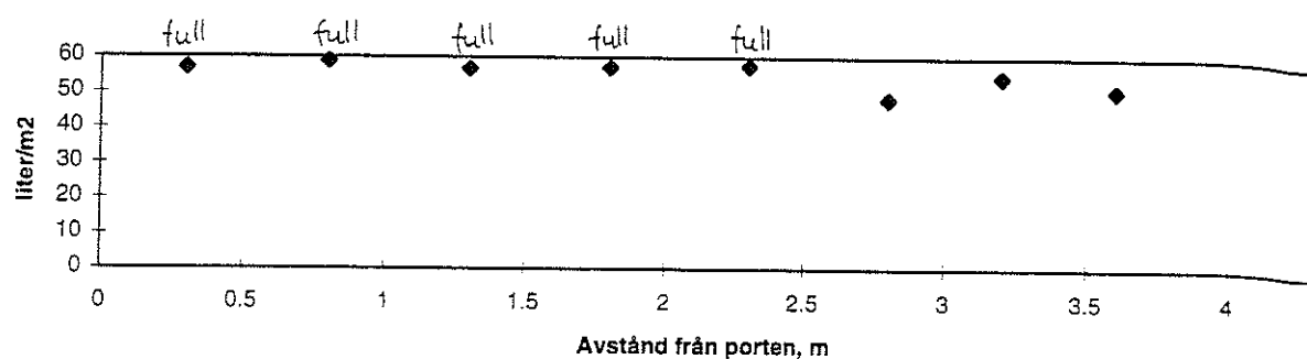
Figur 65. Vattenfördelningen i längsled i golvnivå.
