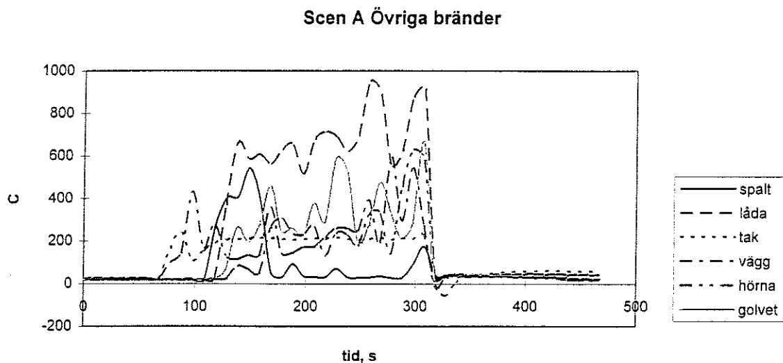
Figur 9. Temperatur övriga bränder.
