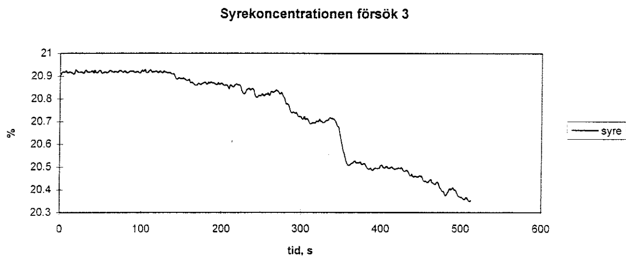
Figur 104. Syrekoncentrationen försök 3.
