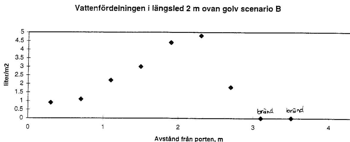
Figur 13. Vattenfördelning längsled 2 m ovan golv
