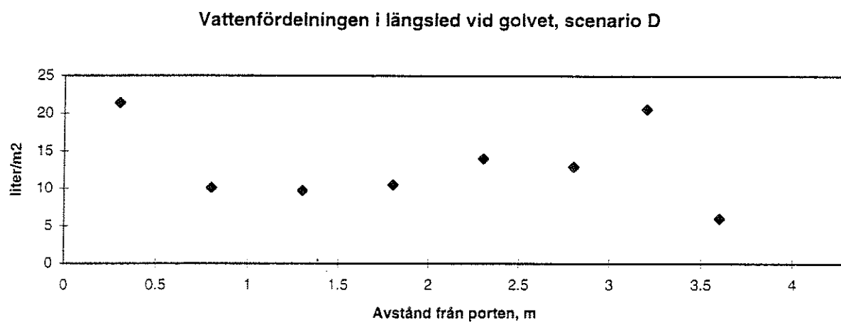
Figur 75. Vattenfördelningen i längsled i golvnivå scenario D.
