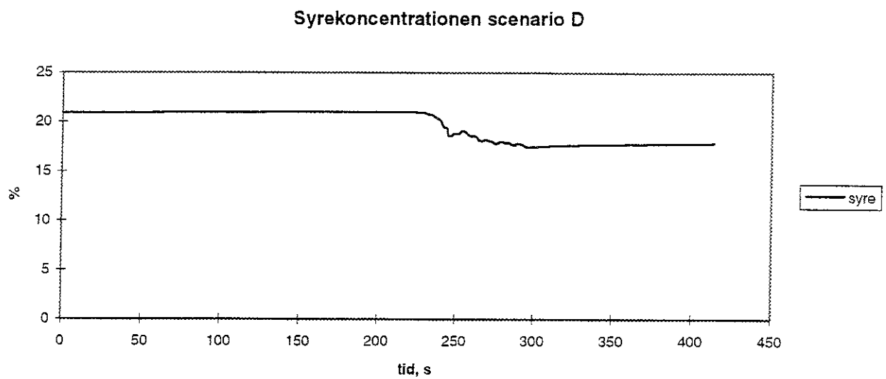
Figur 80. Syrekoncentration scenario D.
