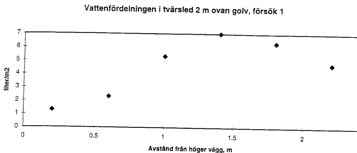
Figur 83. Vattenfördelningen i tvärsled 2 m ovan golv.
