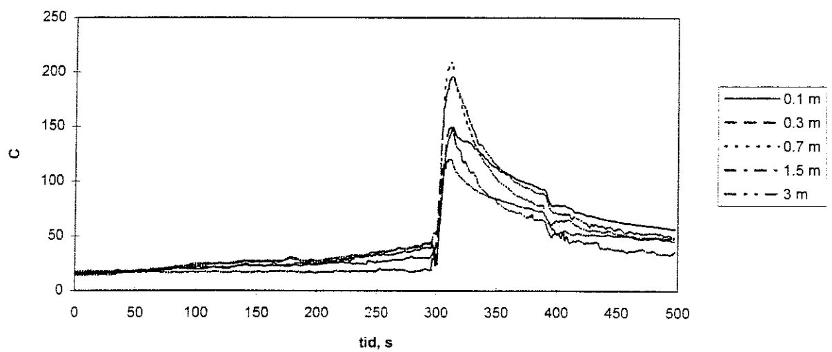
Figur 129. Temperaturträd försök 6.
