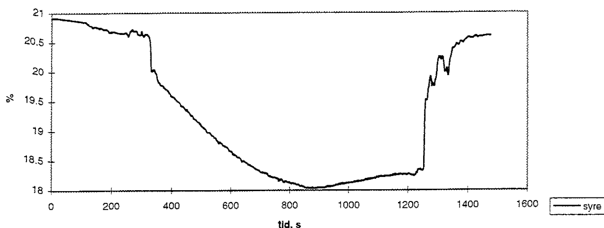
Figur 61. Syrekoncentrationen scenario B.
