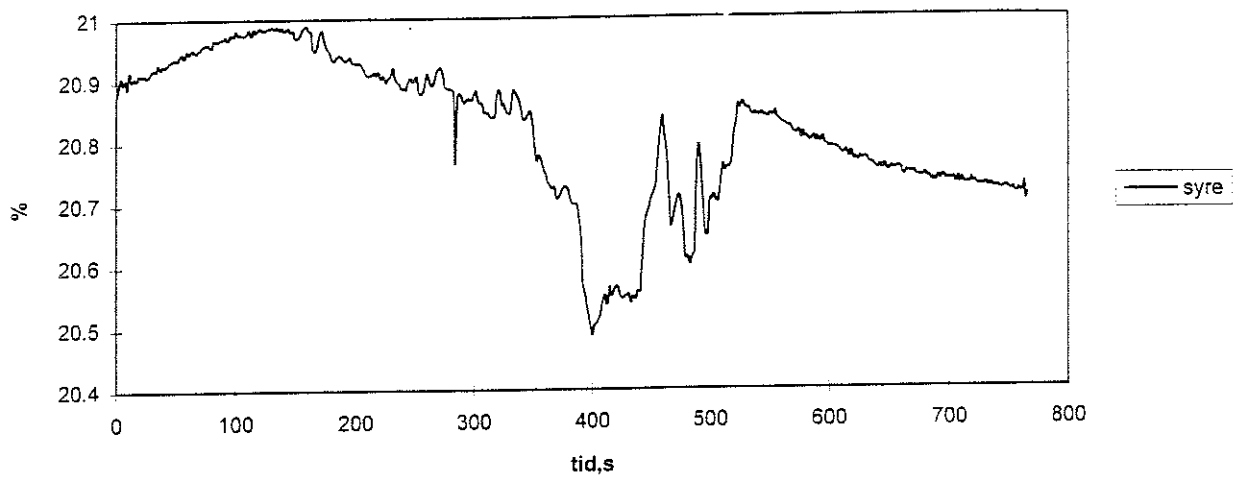
Figur 158. Syrekoncentrationen försök 9.
