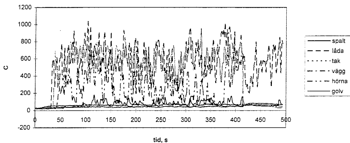
Figur 148. Temperaturen ovan metanolbålen försök 8.
