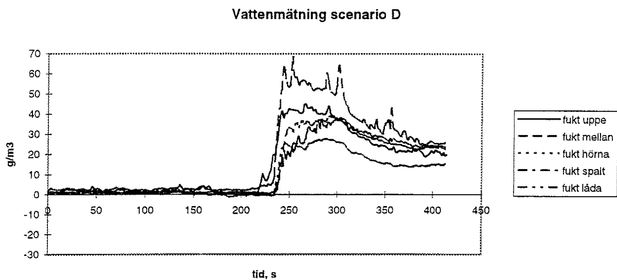
Figur 76. Vattenmätning scenario D.
