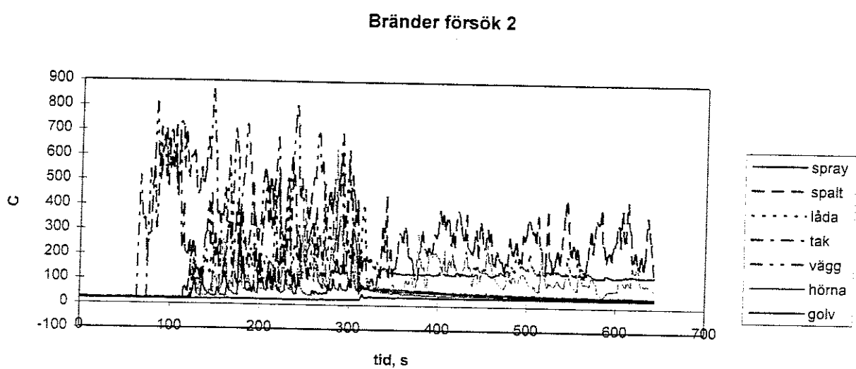
Figur 94. Temperaturen ovan heptanbränderna i försök 2.
