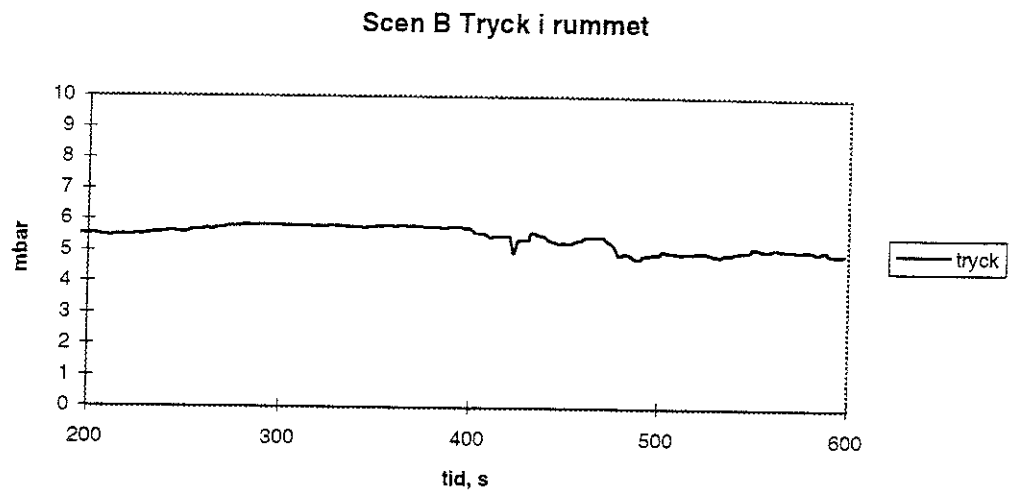
Figur 17. Tryckuppbyggnad i rummet.
