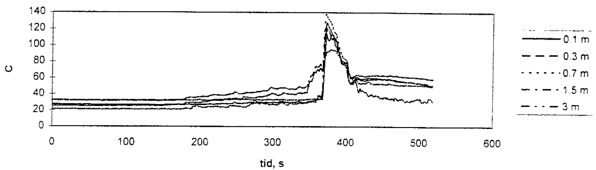
Figur 141. Temperaturträdet försök 7.
