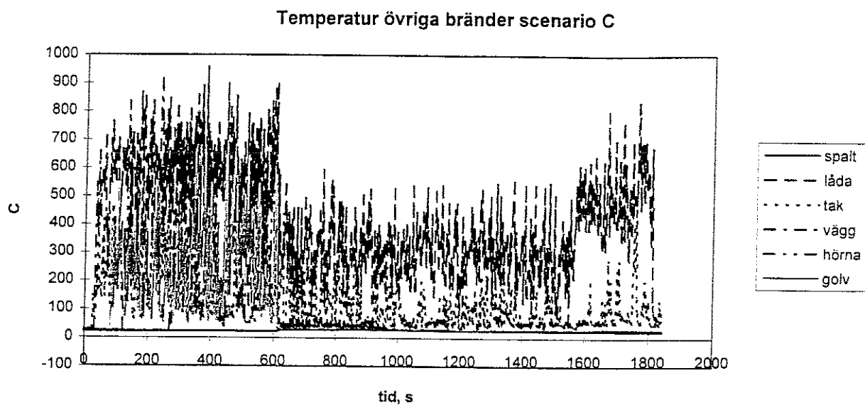
Figur 69. Temperatur övriga bränder scenario C.
