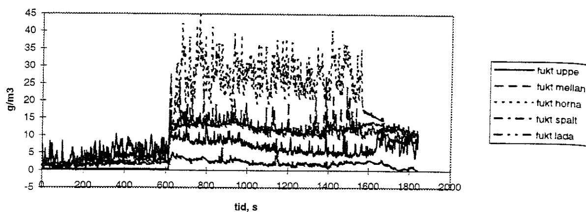
Figur 66. Vattenmätning scenario C.
