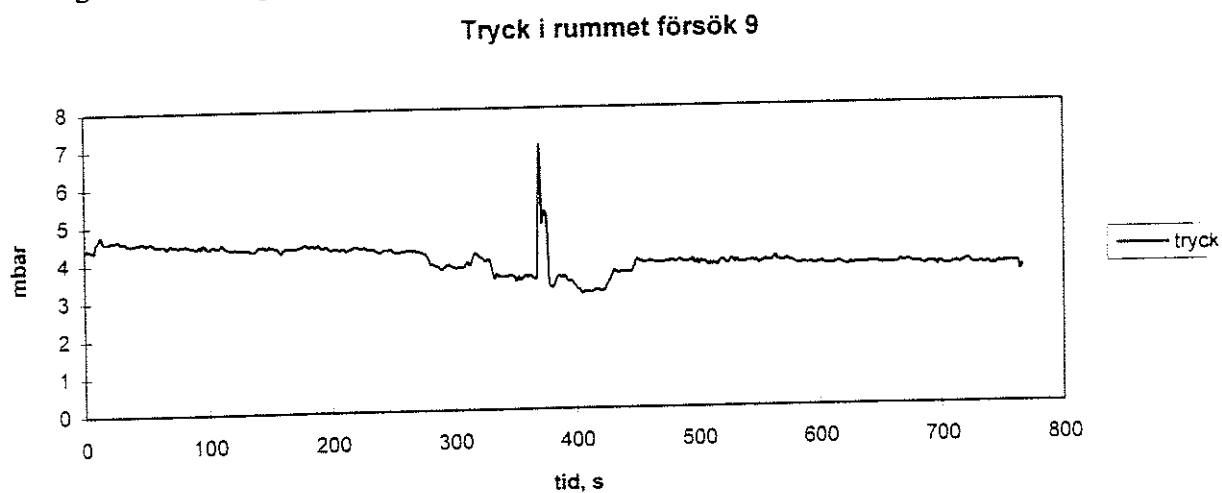
Figur 155. Trycket i rummet försök 9.
