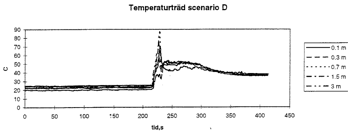
Figur 79. Temperaturträd scenario D.
