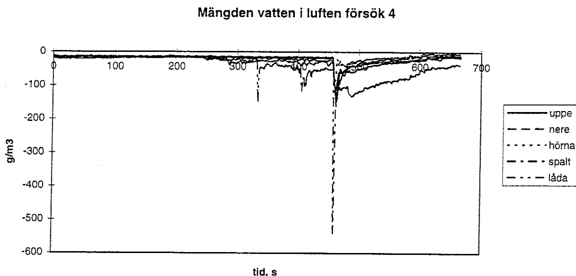
Figur 109. Vatten i luften försök 4
