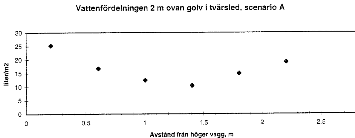
Figur 44. Vattenfördelning 2 m ovan golv i tvärsled.
