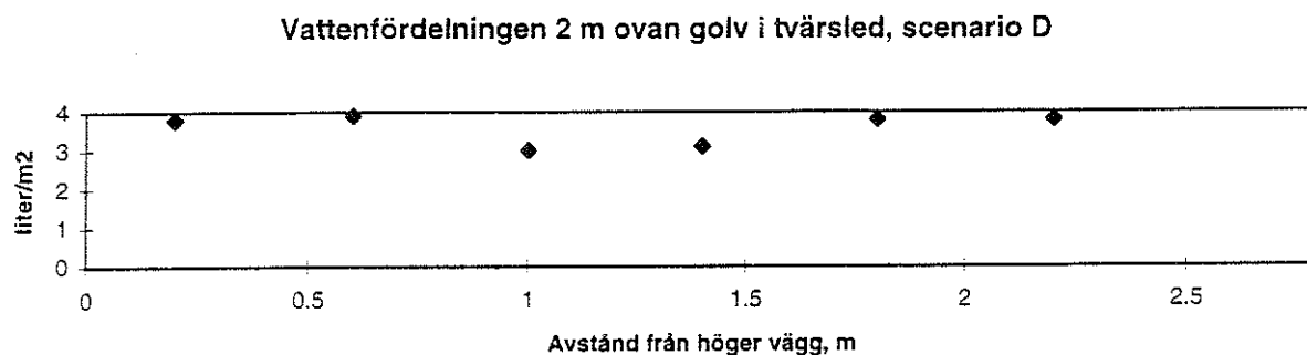
Figur 74. Vattenfördelningen i tvärsled 2 m ovan golv scenario D.
