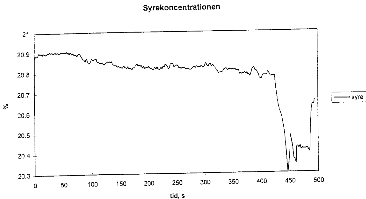
Figur 150. Syrekoncentrationen i rummet försök 8.
