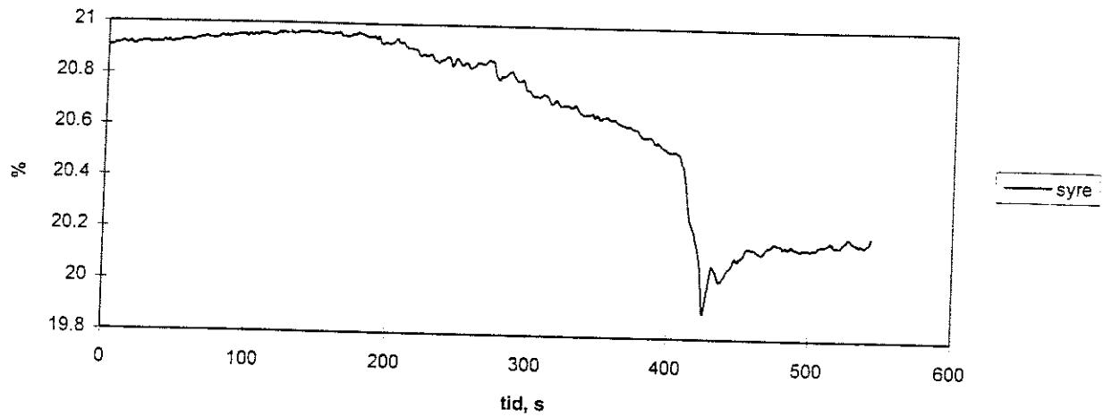
Figur 121. Syrekoncentrationen i rummet försök 5.
