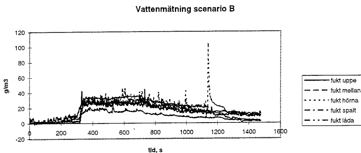
Figur 56. Vattenmätning scenario B.
