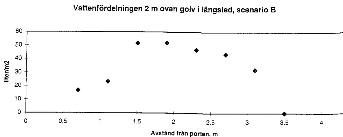
Figur 53. Vattenfördelning i längsled 2 m ovan golv.
