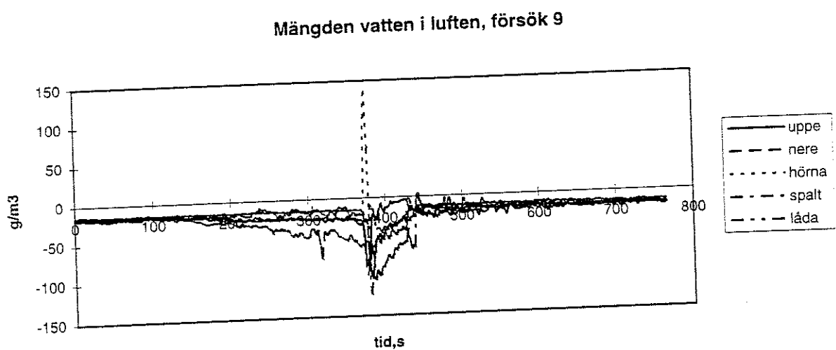
Figur 154. Mängden vatten i luften försök 9.
