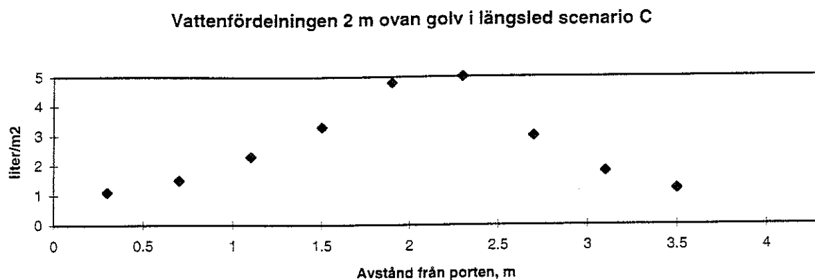
Figur 24 Vattenfördelning längsled 2 m ovan golv
