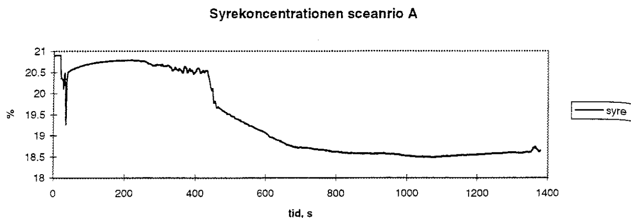
Figur 51. Syrekoncentration scenario A.
