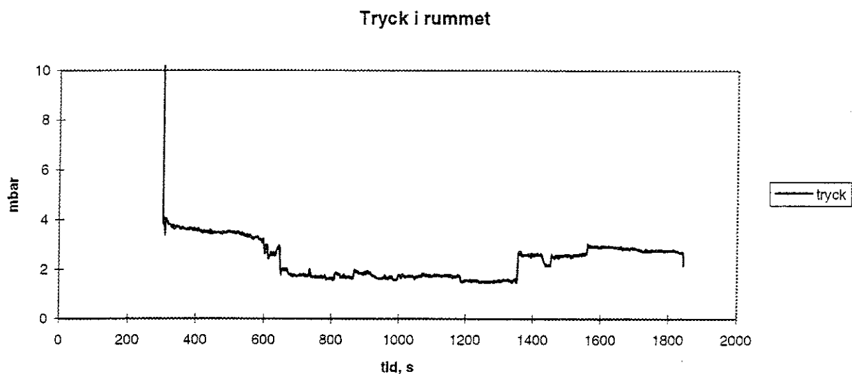
Figur 67. Tryck i rummet scenario C.
