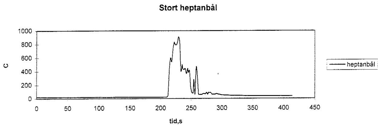
Figur 78. Temperatur ovan branden scenario D.
