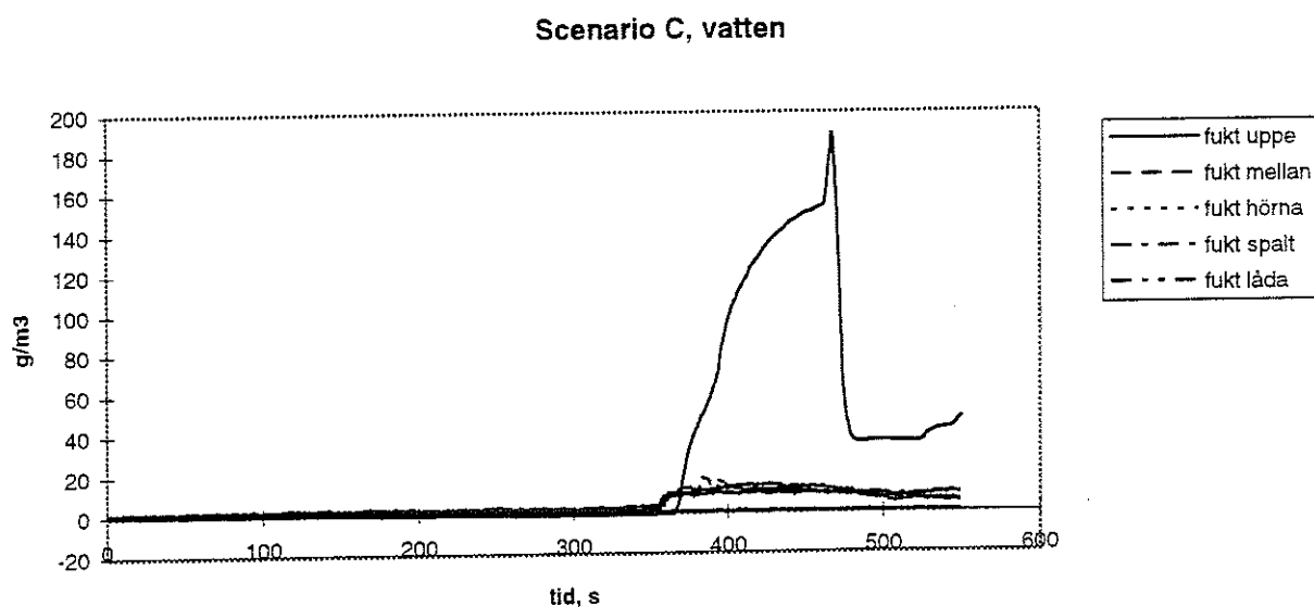
Figur 26. Vattenmätning scenario C
