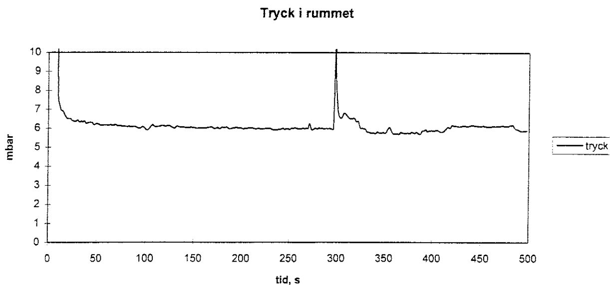
Figur 126. Tryck i rummet försök 6.
