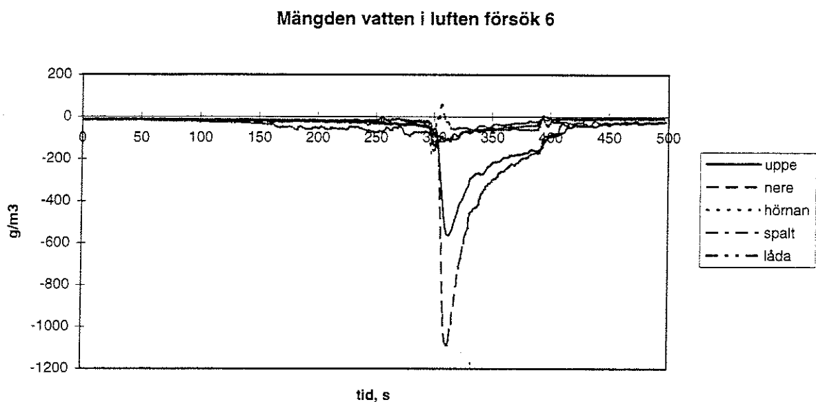
Figur 125. Vatten i luften försök 6.
