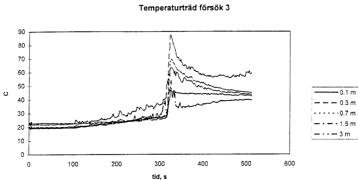
Figur 103. Temperaturträd försök 3.
