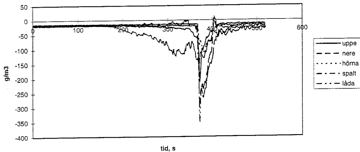
Figur 137. Vattenmängden i luften försök 7.
