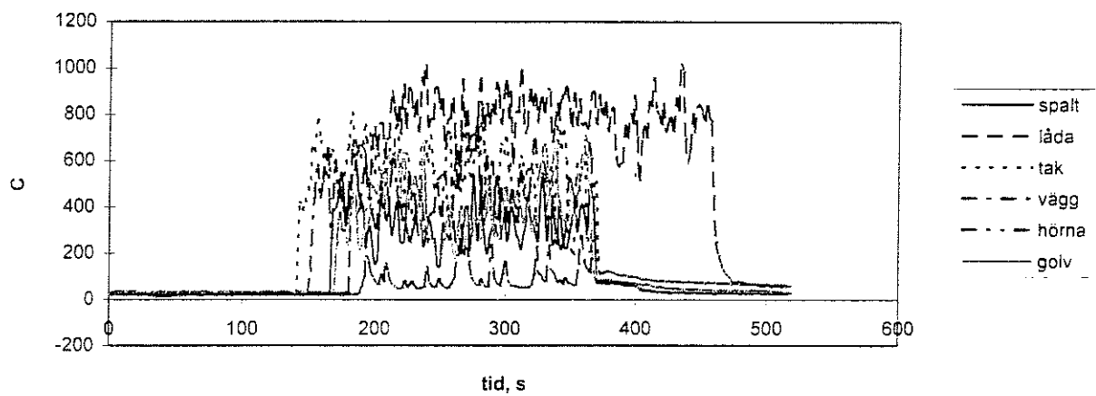
Figur 140. Övriga bränder försök 7.
