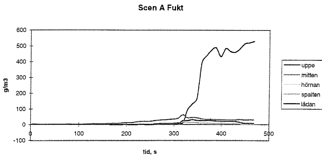
Figur 6. Fuktmätning scenario A
