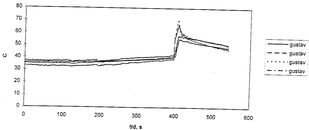
Figur 122. Hudtemperaturen på Gustav försök 5
