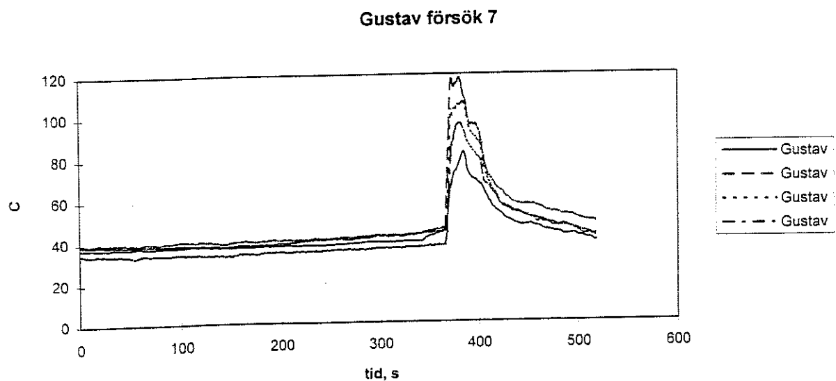
Figur 143. Hudtemperaturen på Gustav försök 7.
