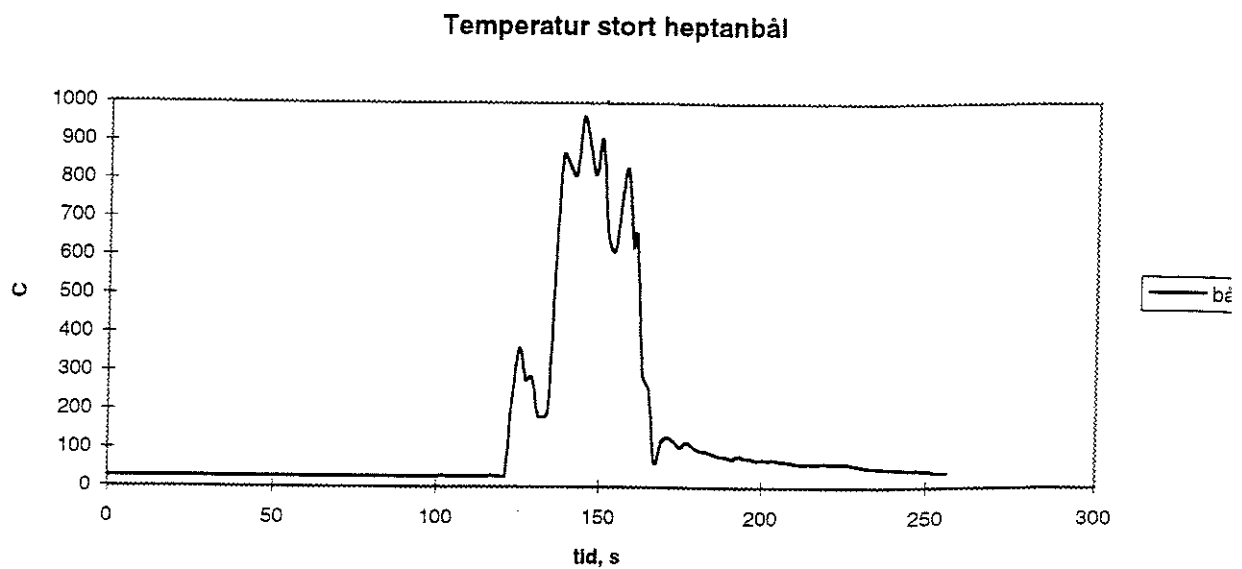
Figur 38. Temperatur ovan branden, scenario D.
