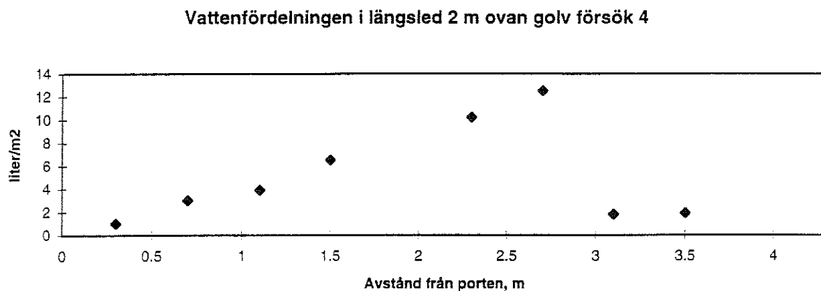
Figur 107. Vattenfördelningen i längsled 2 m ovan golv försök 4.
