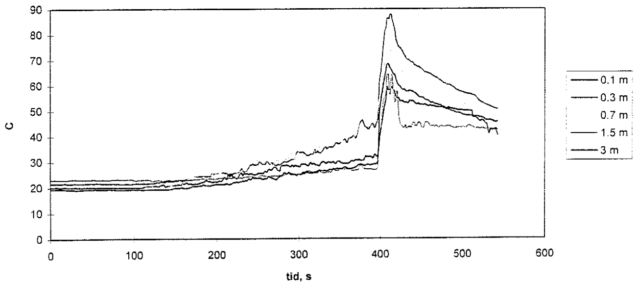
Figur 120. Temperaturträd försök 5.
