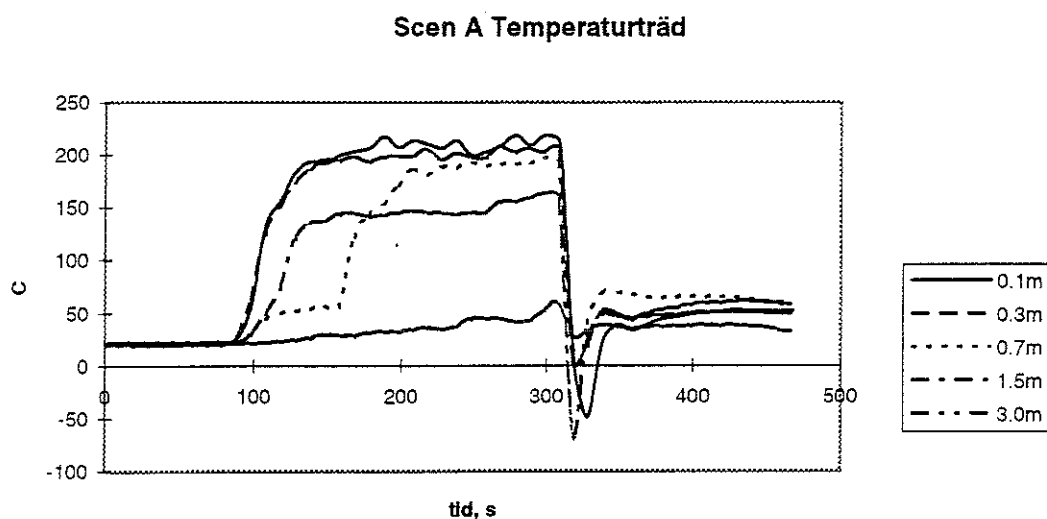
Figur 10. Temperaturträd.
