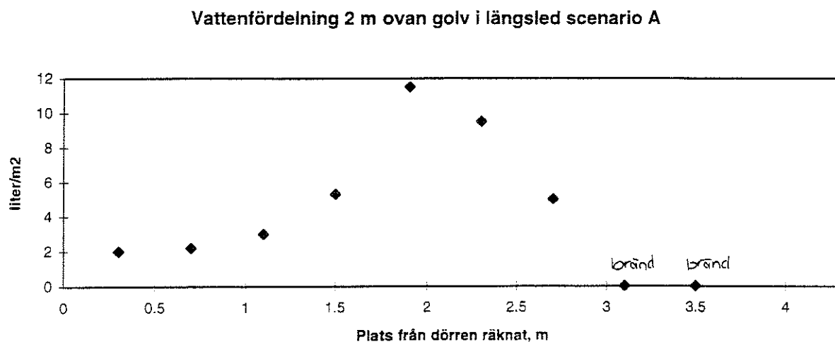
Figur 4 Resultat av muggvägning längs containern 2 m ovan golv
