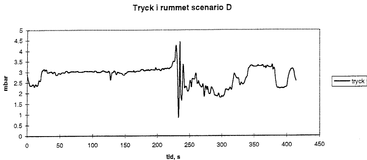
Figur 77. Tryck i rummet scenario D.
