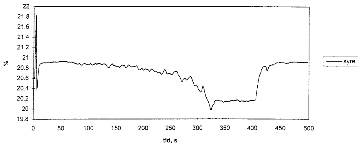
Figur 130. Syrekoncentrationen i rummet försök 6.
