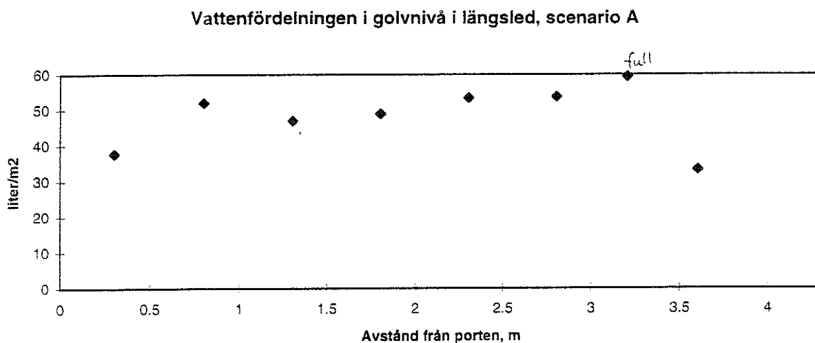
Figur 45. Vattenfördelning i längsled i golvnivå.
