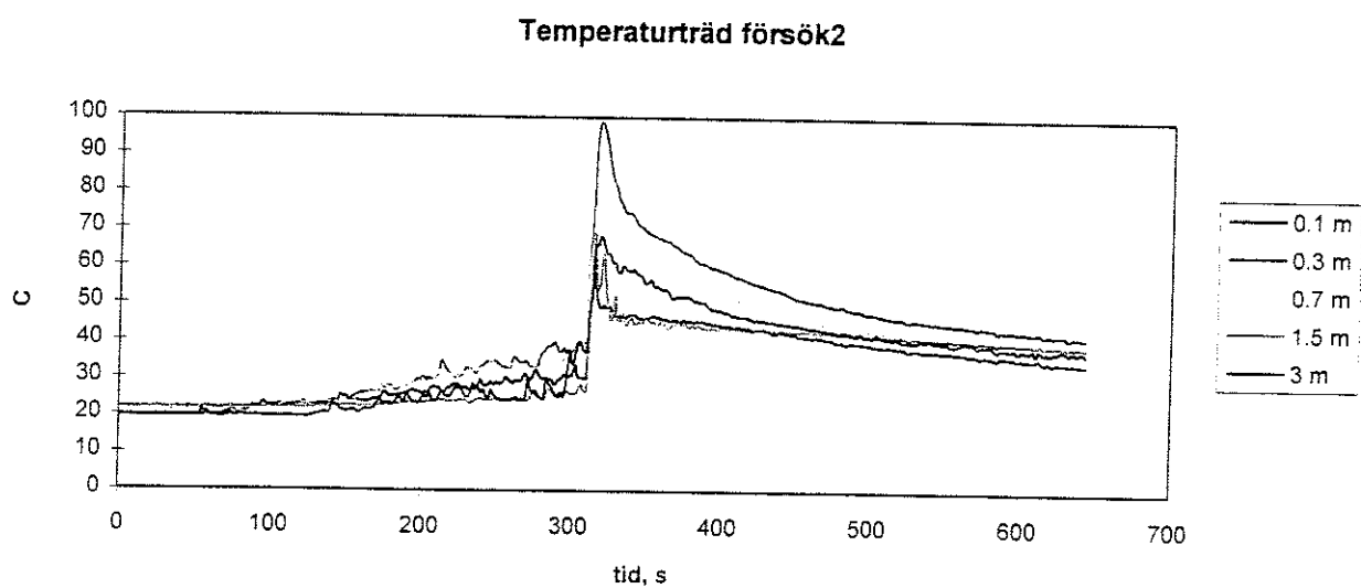
Figur 95. Temperaturträd försök 2.
