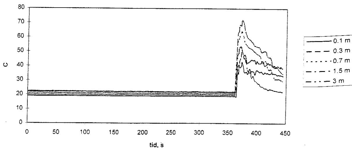
temperatur försök 1
