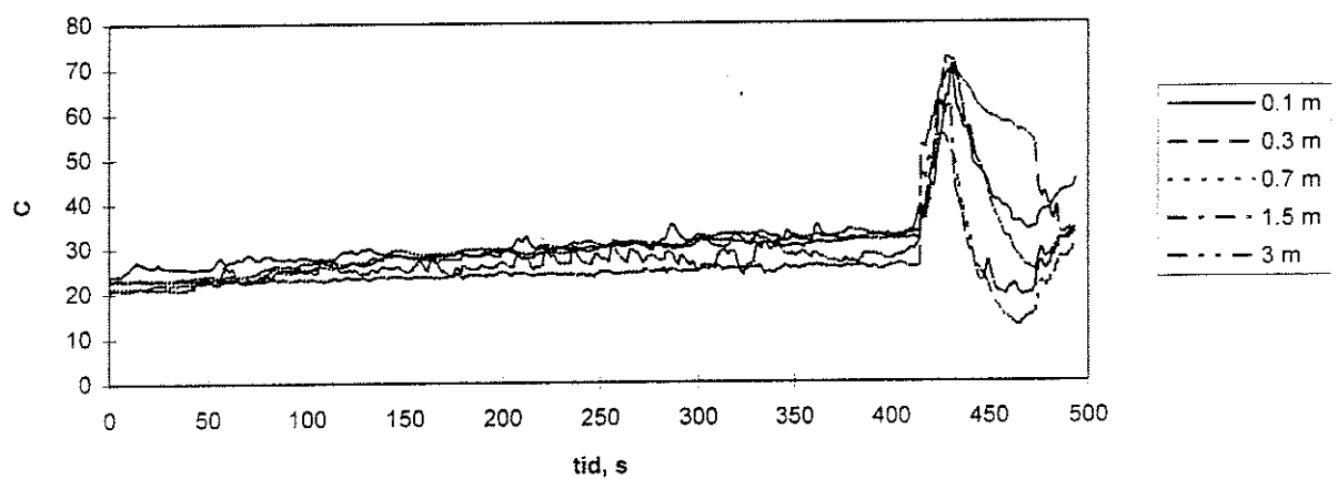
Figur 149. Temperaturträdet försök 8.
