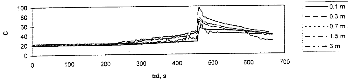
Figur 112. Temperaturträd försök 4
