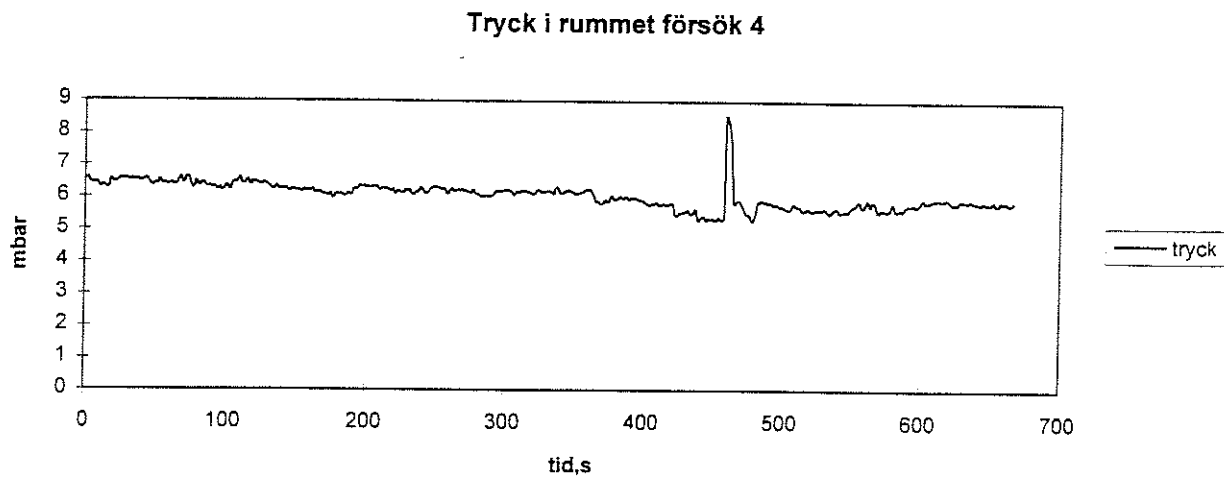
Figur 110. Trycket i rummet försök 4.
