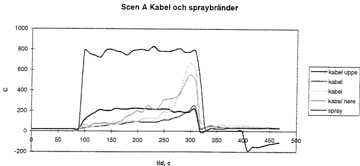
Figur 8. Temperatur kabel och spraybrand
