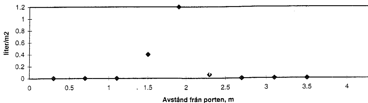
Figur 115. Vattenfördelningen 2 m ovan golv i längsled.
