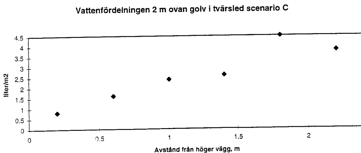
Figur 23. Vattenfördelning tvärsled 2 m ovan golv scenario C.
