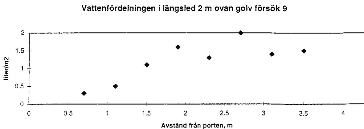
Figur 152. Vattenfördelningen 2 m ovan golv i längsled försök 9.
