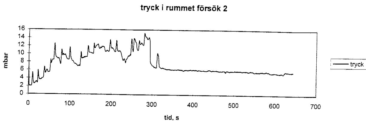
Figur 93. Tryck i rummet försök 2
