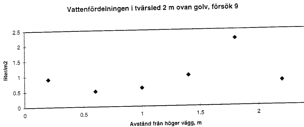
Figur 153. Vattenfördelningen 2 m ovan golv i tvärsled försök 9.
