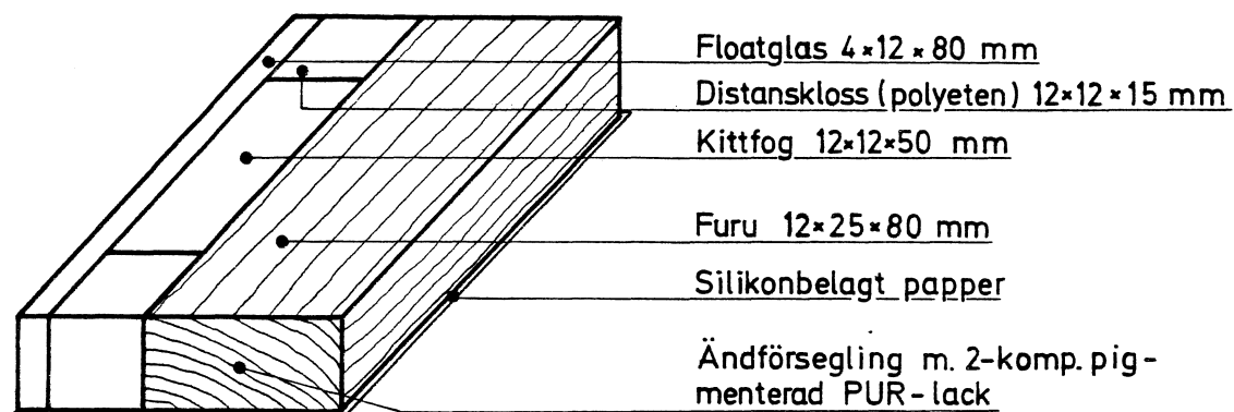
FIGUR 4.1 Laborieprovkropparnas utformning.
