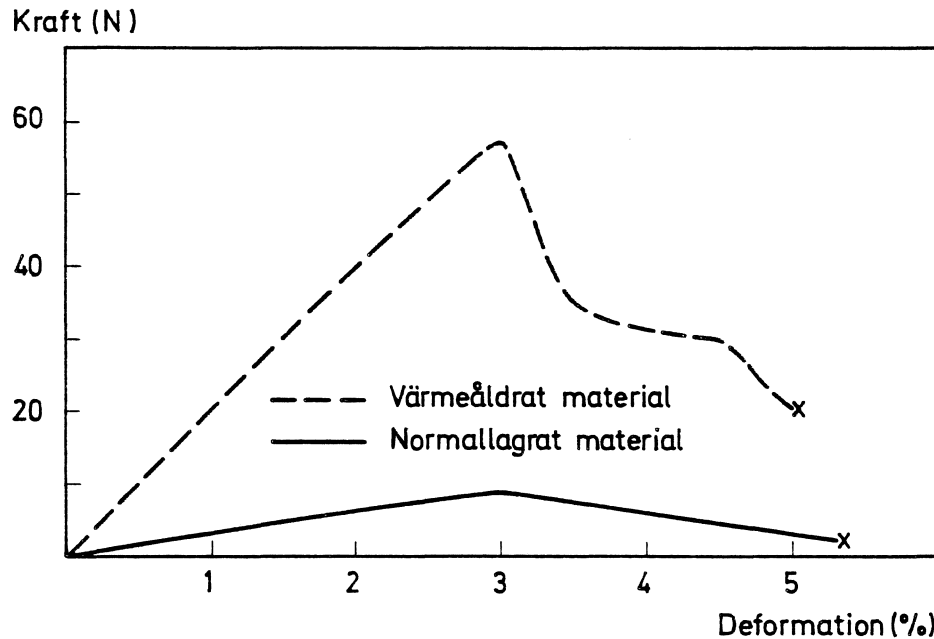
FIGUR 6.2 Exempel på samband mellan kraft och deformation för kitt nr 8 mellan glas och vacuumimpregnerat trä.
