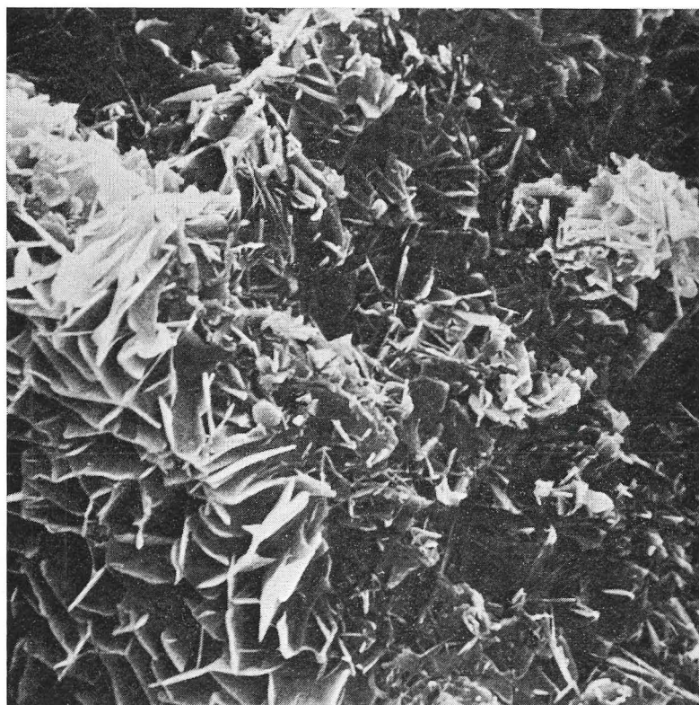
Fig. 9. Gasbetong-struktur sett i scanning-elektronmikroskop. I nedersta vänstra hörnet syns strukturen i en blåsas yta. Den övriga delen av bilden visar en brott-yta i en porvägg. De enskilda kornen är kristaller av hydratiserade kalciumsilikater. (Södertälje Siporex).
