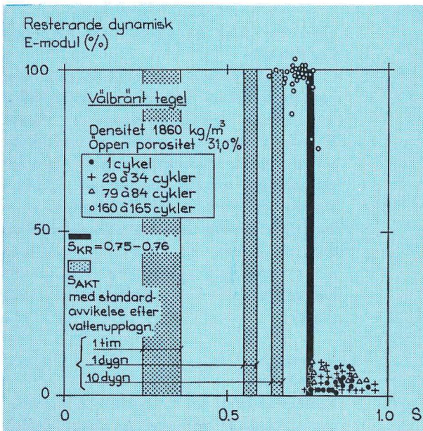
Fig. 3. Kritisk ( S_{KR} ) och aktuell ( S_{AKT} ) vattenmättnadsgrad hos välbränt tegel.
