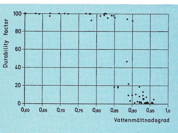
Fig. 1. Vattenmättnadsgradens inverkan på "durability factor" enl. Whiteside och Sweet.
