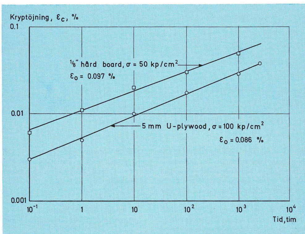
Fig. 6. Krypcurvorna för 5 mm U-plywood och 1/8" hård board, enl. Lundgren. Spänningarna avser dragbelastning. Krypcurvorna är räta linjer i det dubbellogaritmiska diagrammet.
