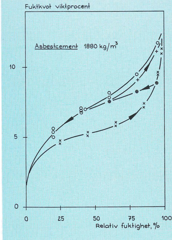
Fig. 16. Absorptions- och desorptionsisotermier för asbestcement, densitet 1880 \text{ kg/m}^3 .
