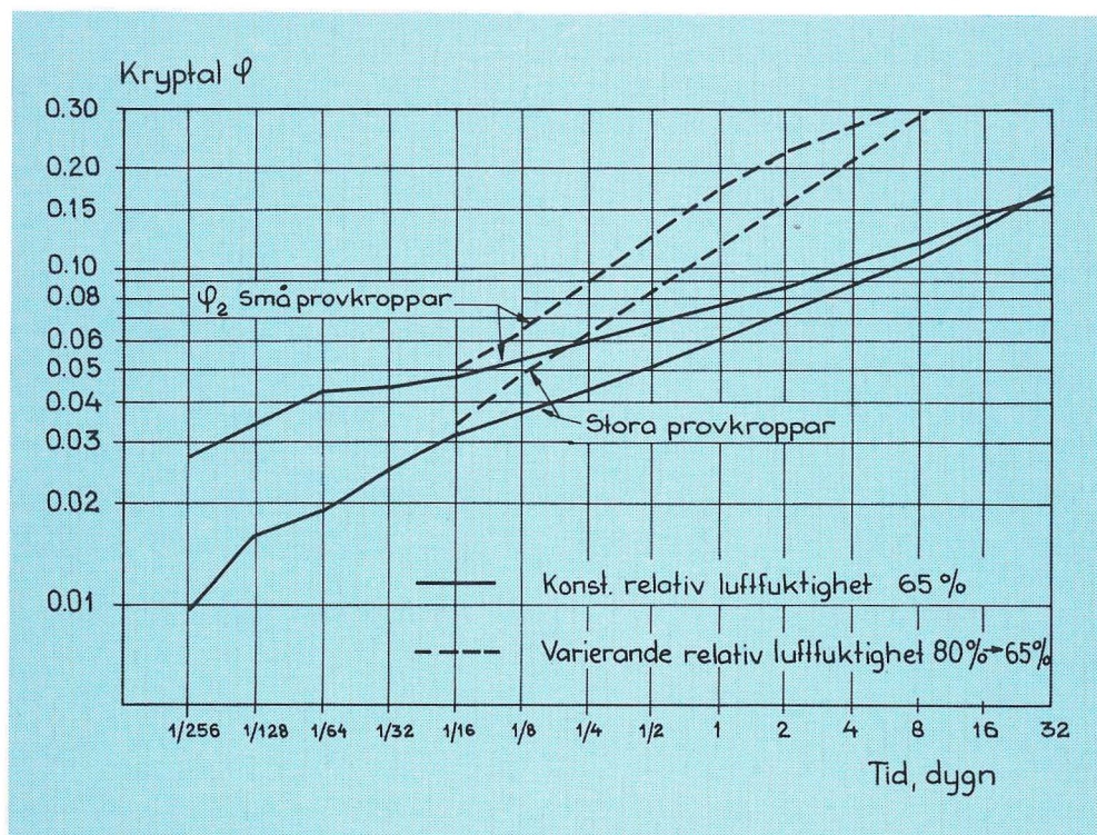
Fig. 12. Resultat av krypförsök med konstruktionsträ och helrent virke. Kryptal som funktion av belastningstid. Heldragna kurvor: Konstant klimat 65 % r.f. Streckade kurvor: Uttorkning 80 % till 65 % r.f.
