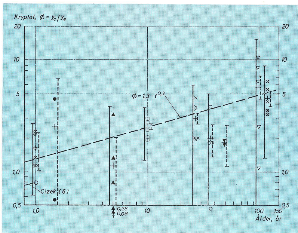
Fig. 11. Långtidsdeformationer i träbjälklag. Kryptal som funktion av belastningstid.
