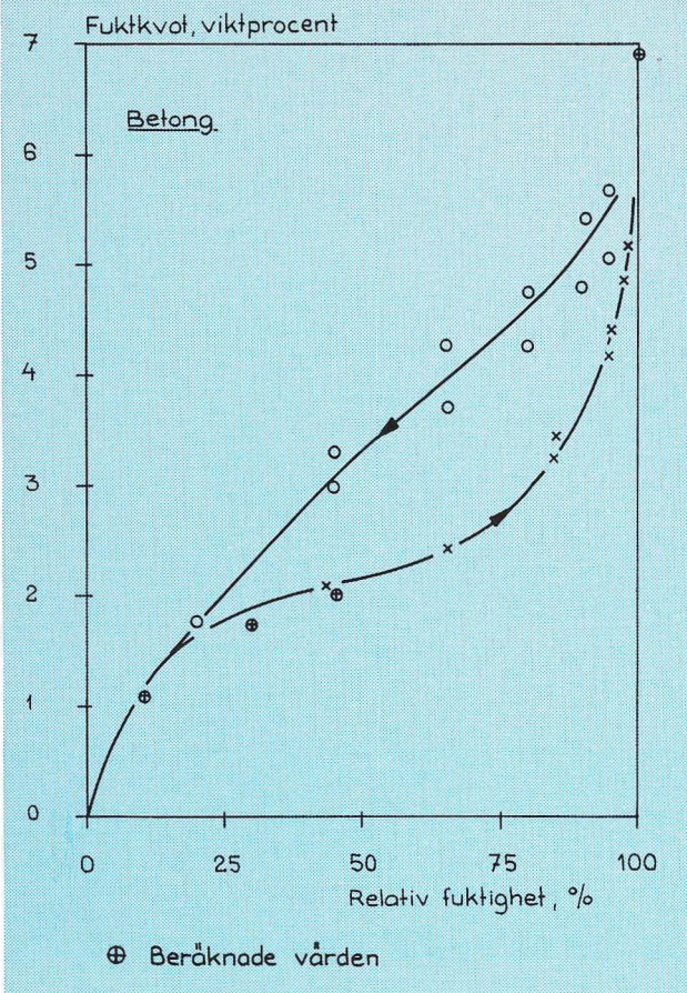
Fig. 18. Absorptions- och desorptionsisotermier för betong ( C = 400 \text{ kg/m}^3 , v_{ct} = 0,55 , w_n/C = 0,23 ) med beräknade värden inlagda.
