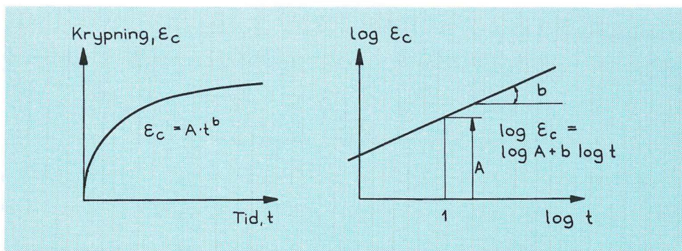
Fig. 5. Krypfunktion \varepsilon_c = A \cdot t^b bildar en rät linje i log-log-diagram.
