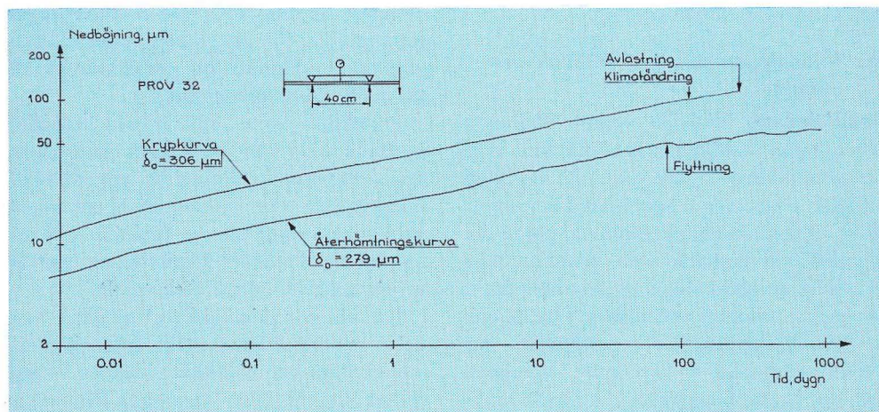
Fig. 7. Krypkurva och återhämningskurva för Dalby Siporex, nr 32. Vattenmättad. Spänning 4 kp/cm 2 Böjbelastning.
