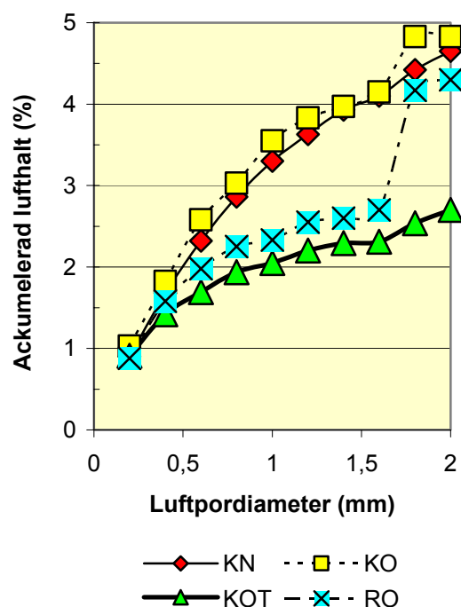
Figur 7.1 – Ackumulerad lufthalt vs luftpordiameter för betonger enligt Appendix 7 [25]. K = kalkstensfiller, N = ny blandningsordning (filler sist), O = ordinarie, R = normal betong (SKB i övrigt), T = 5.5 m gjuttryck (0.25 m i övrigt).
