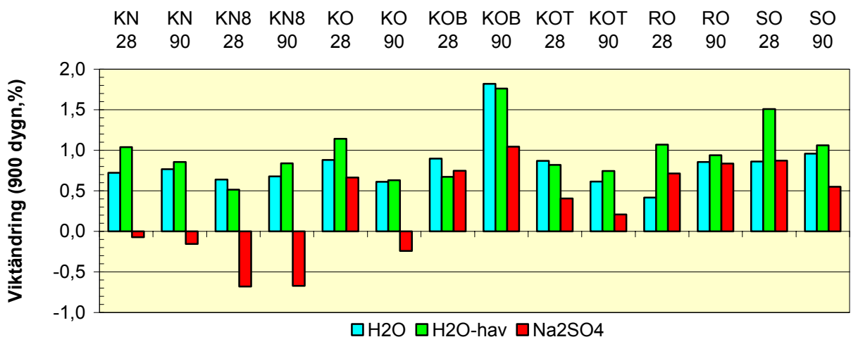
Figur 9.3 - Viktändring efter 900 dygns exponering i destillerat vatten, havsvatten och sulfat. Beteckningar: B = ökad fillermängd, K = Limus 40; N = ny blandningsordning (filler sist); O = ordinarie blandningsordning (filler först); R = referens (VB), S = Limus 15; T = 5.5 m hydrostatiskt tryck i stället för 0.23 m; II = andra; 8 = 8% lufthalt.
