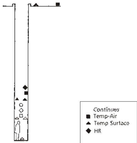
Fig. 3.13 Coupe montrant l'emplacement des points de mesure (continues et momentanées) au quartier traditionnel Seffarine
