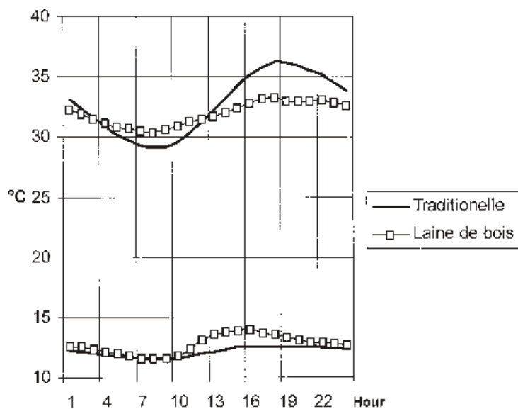
Fig. 5.19 Toiture isolée comparée à une toiture traditionnelle (bâtiment ventilé). Température du plafond en janvier (à gauche) et en juillet (à droite)
