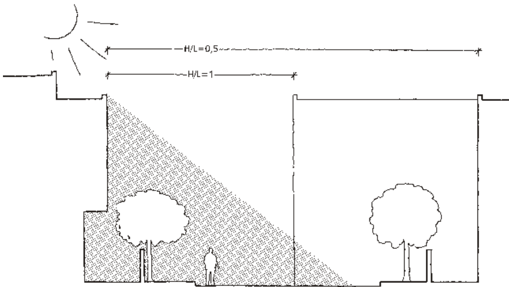
Fig. 3.29 Calcul de la longueur de l'ombre : canyon urbain orientation est-ouest en février à 9h et à 15h
