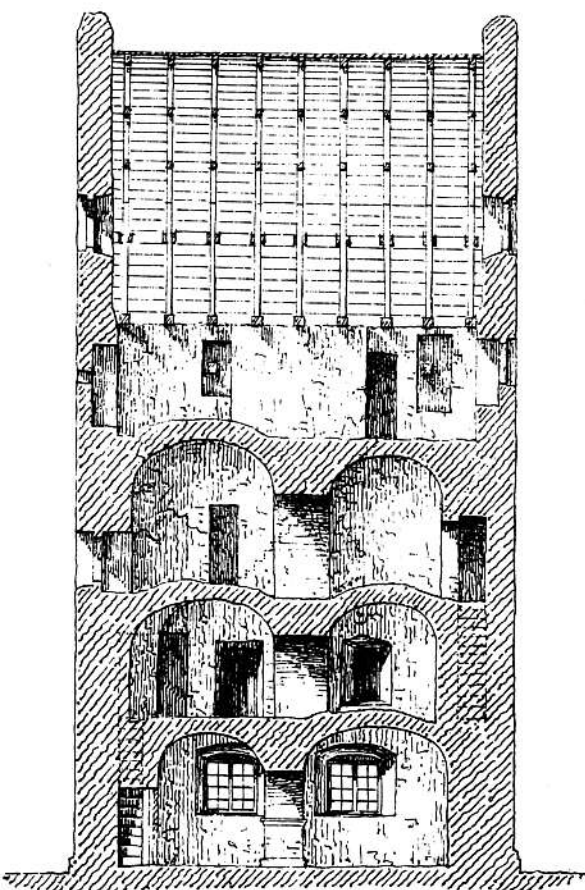
Fig. 4. Ibs kirkes vesttårn i tværsnit set fra øst. Skala ca. 1:200. Tegning i Holm 1878.
