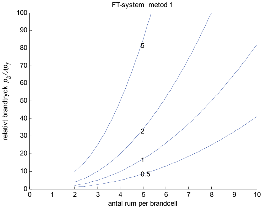
Figur 3.3 Relativt brandtryck p_b/\Delta p_f för olika antal rum n och olika kvot \Delta p_t/\Delta p_f .
