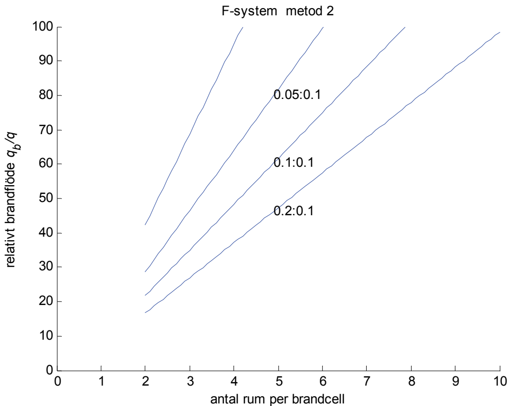
Figur 2.7 Relativt brandflöde q_b/q för rumantal n , tryckfallskvot \Delta p_l/\Delta p_f och \Delta p_s/\Delta p_f = 0.1 .
