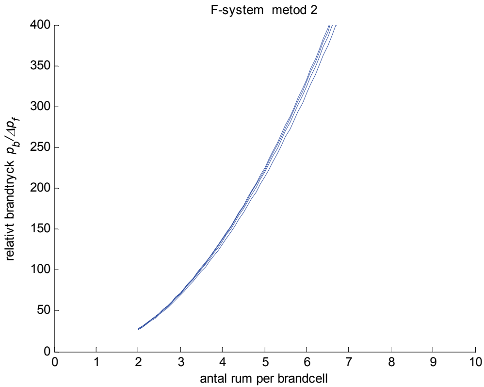
Figur 2.6 Relativt brandtryck p_b/\Delta p_f för rumantal n , tryckfallskvot \Delta p_l/\Delta p_f och \Delta p_s/\Delta p_f = 0.1 .
