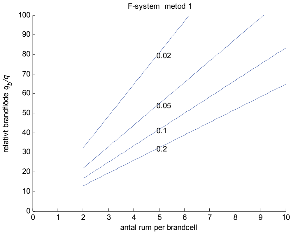
Figur 2.4 Relativt brandflöde q_b/q för olika antal rum n och tryckfallskvot \Delta p_l/\Delta p_f .
