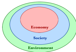
Figur 3: Här illustreras att såväl social som ekonomisk ”sustainability” ska ses som underordnat den ekologiska (Scott Cato 2009).
