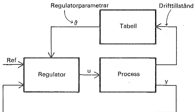
Fig. 3.15. Blockschemata för regulator med parameterstyrning. Regulatorns parametrar \vartheta bestäms som funktioner av drifttillståndet genom tabelluppslagning och interpolation.
