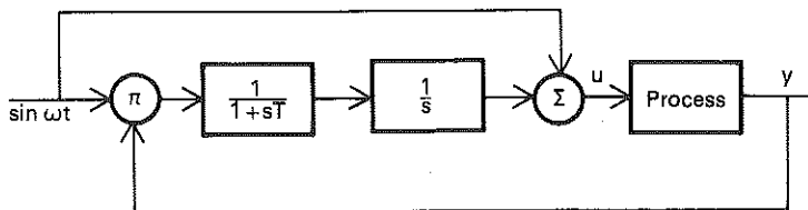
Fig. 3.12. En extremalsökande regulator enligt Draper och Li.
