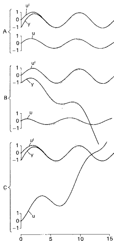
Fig. 4.4. Simulering av systemet i fig. 4.2. I fall A är processen och inversen stabila ( a = 1, b = 2 ). Efter en transient kommer y och u^I att överensstämna. I fall B ( a = -0,2, b = 2 ) är processen instabil. Processens utsignal y kommer då att växa utan gräns. I fall C ( a = 1, b = -0,2 ) är processen stabil men inversen instabil. Processens insignal u växer då som \exp -bt . Nollstället s = -b blockerar emellertid denna komponent av insignalen och y överensstämmer med u^I efter en transient.
