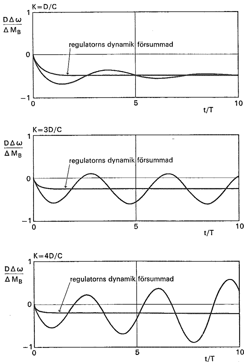
Fig. 2.9. Visar vinkelhastighetsförändringen \Delta \omega efter en ökning av belastningen för en ängmaskin med proportionell återkoppling med olika värden på regulatorns förstärkning. Regulatorns parametrar har valts så att \beta T = 1 och \zeta = 0,5 . Figuren visar även vad som händer då regulatorns dynamik försummas i analysen.
