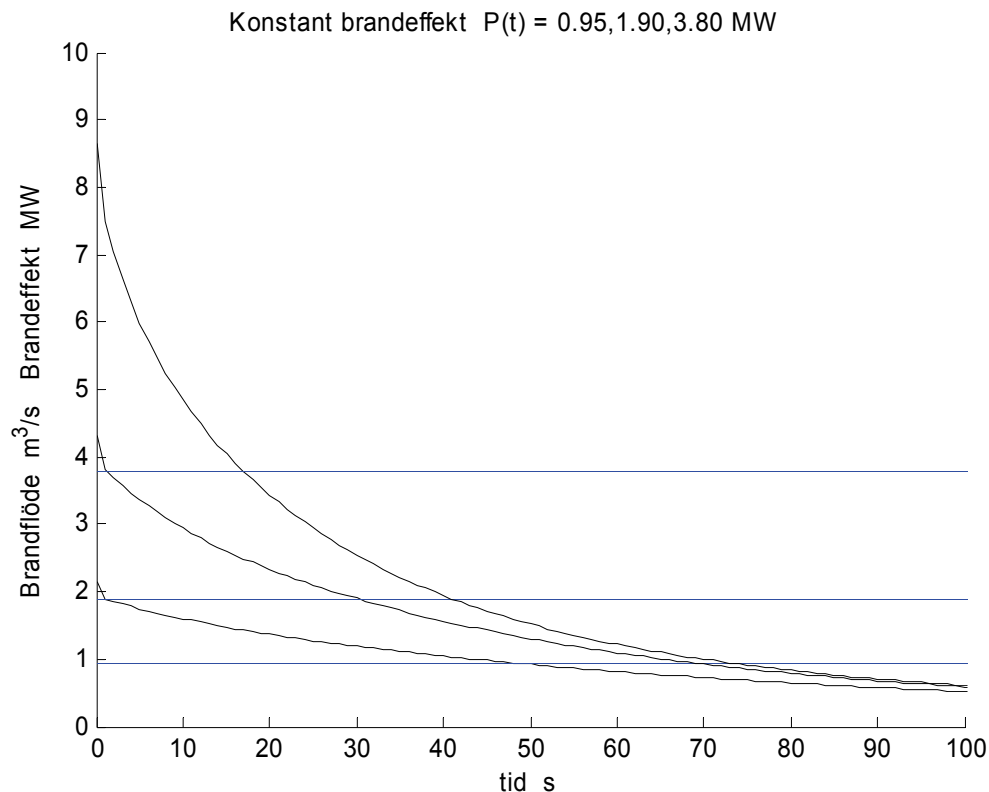
Figur 3.16 Brandflöde och brandeffekt för olika konstanta brandeffekter.
