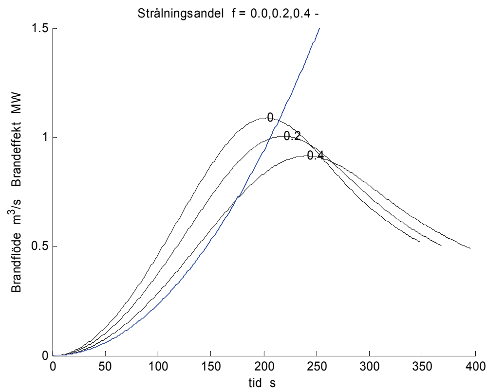
Figur 3.10 Brandflöde och brandeffekt för olika strålningsandel f = 0.0, 0.2 och 0.4 .
