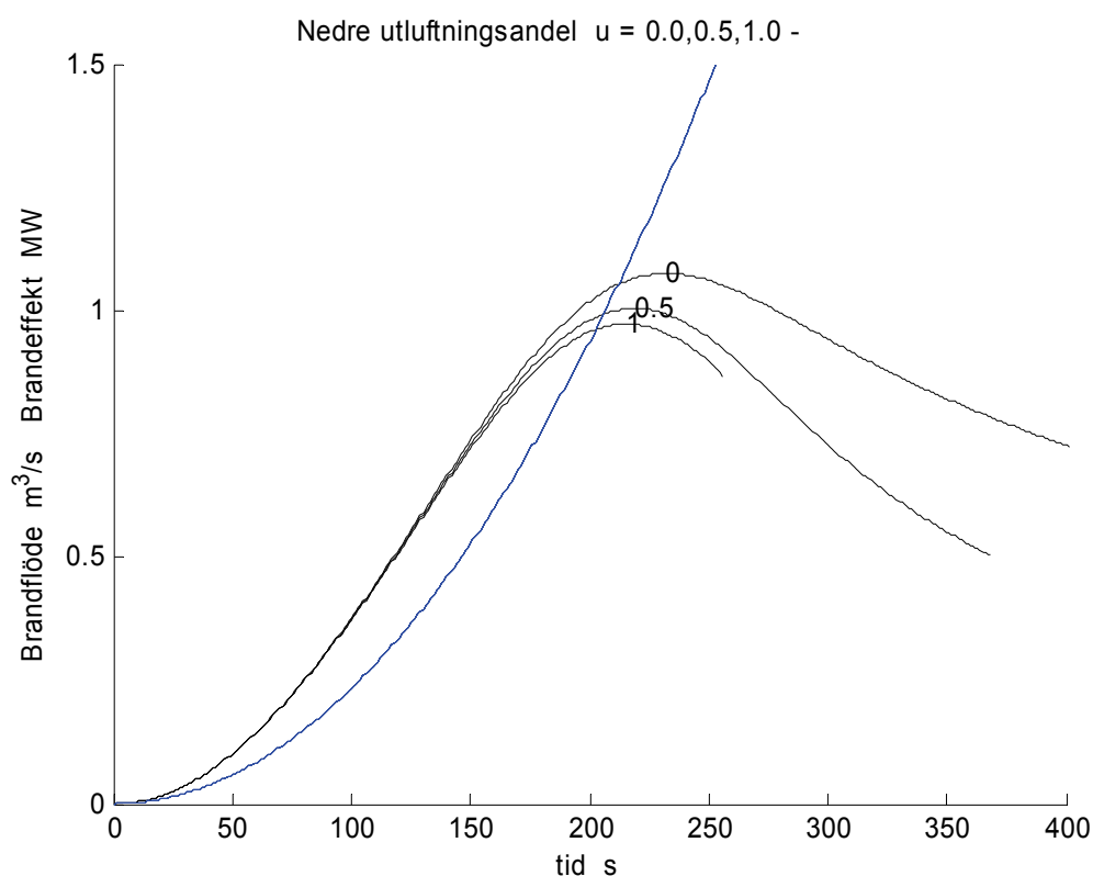
Figur 3.9 Brandflöde och brandeffekt olika nedre utluftsandel u = 0.0, 0.5 och 1.0 .
