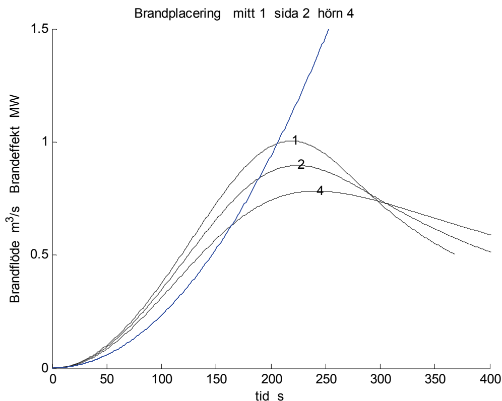
Figur 3.12 Brandflöde och brandeffekt för olika brandplacering mitt, sida och hörn med motsvarande plymparameter m = 1, 2 och 4 .
