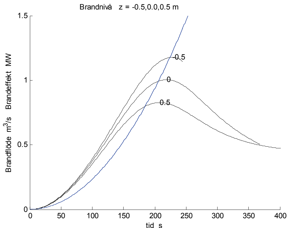
Figur 3.13 Brandflöde och brandeffekt för olika brandnivå z = -0.5, 0.0 och 0.5 m.
