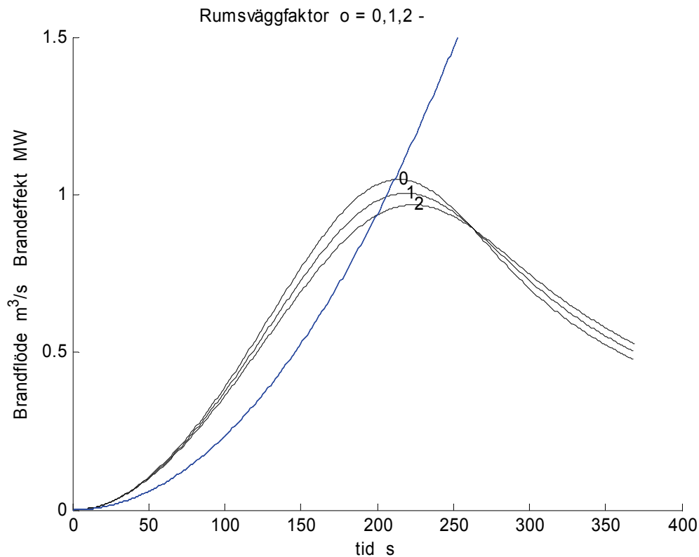
Figur 3.5 Brandflöde och brandeffekt för olika rumsväggfaktor \sigma = 0, 1 och 2 .
