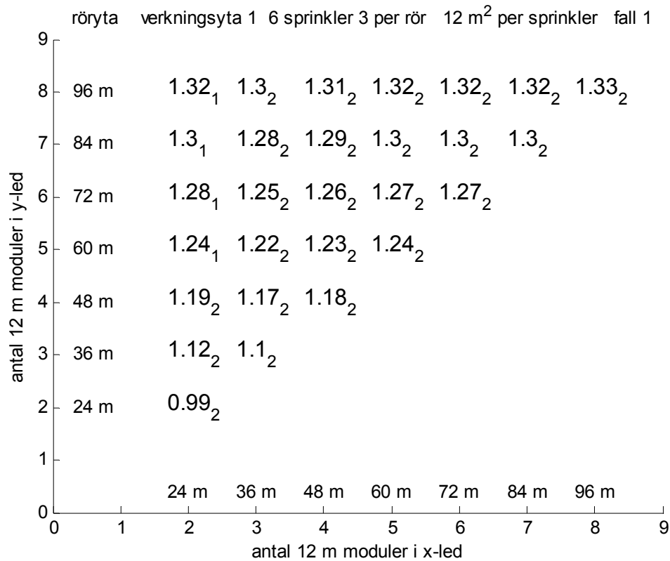
Figur 4.3 Relativ rörytkvot mellan grenrör och gridrör för verkningsyta 1.
