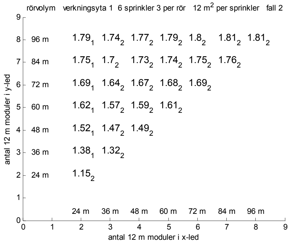
Figur 4.4 Relativ rörvolymkvot mellan grenrör och gridrör för verkningsyta 1.
