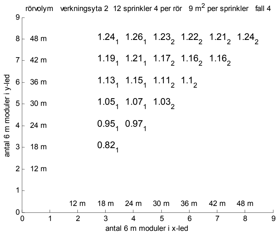
Figur 4.14 Relativ rörvolymkvot mellan grenrör och gridrör för verkningsyta 2.
