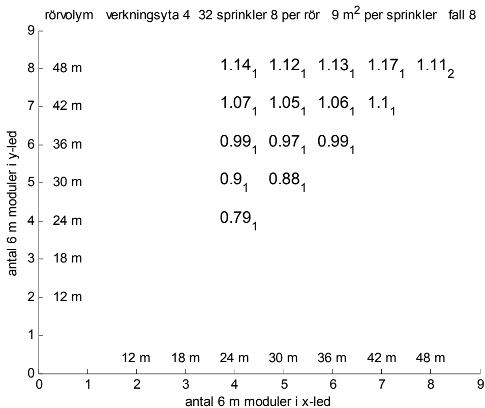
Figur 4.18 Relativ rörvolymkvot mellan grenrör och gridrör för verkningsyta 4.
