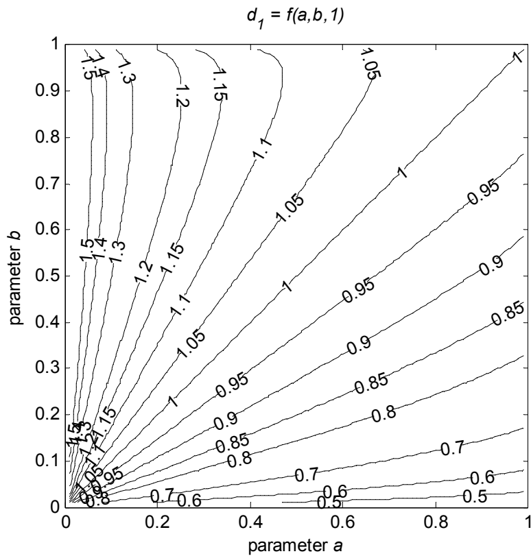
Figur 2.6 Diameterfunktion d_l = f(a, b, 1) för lägsta röryta.
