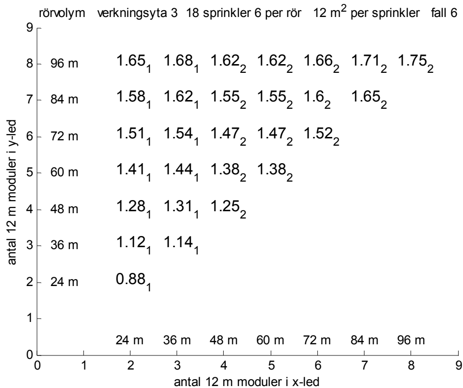
Figur 4.8 Relativ rörvolymkvot mellan grenrör och gridrör för verkningsyta 3.
