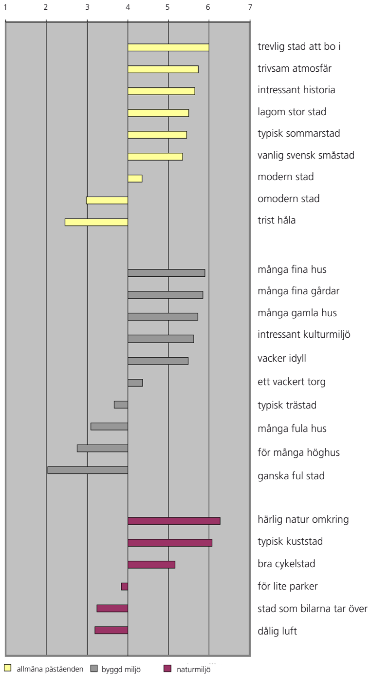
Karlsхамns identitet, generella resultat
